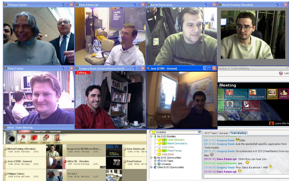
Fig. 10: EVO
