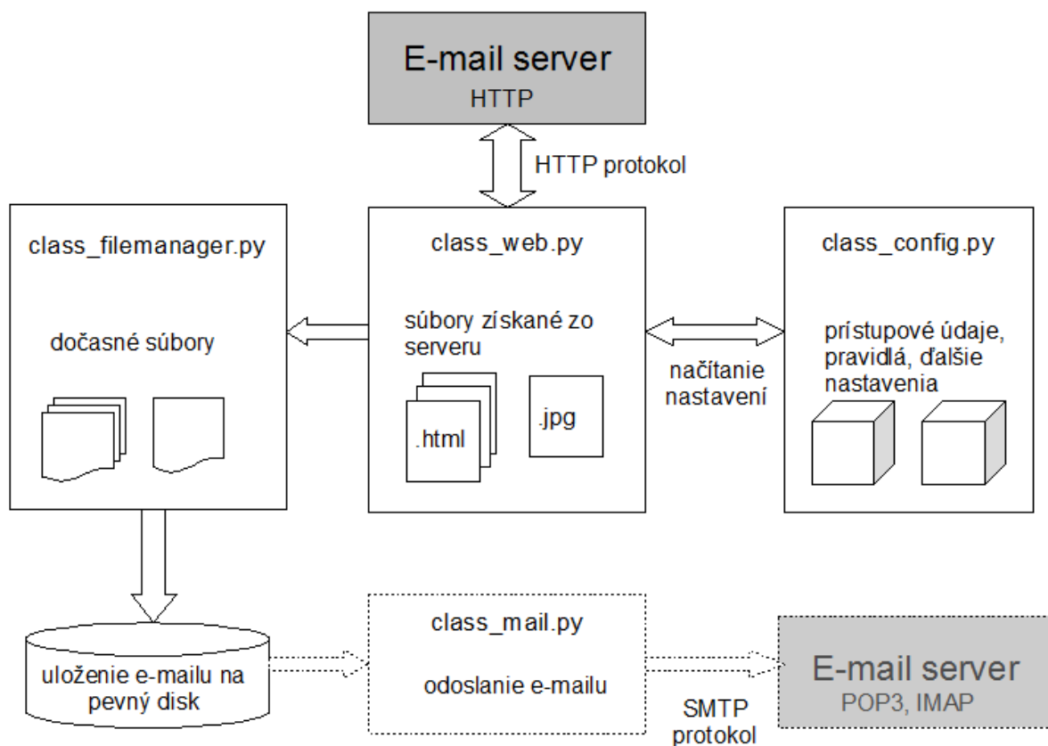
Obrázok 5.1: schéma aplikácie
