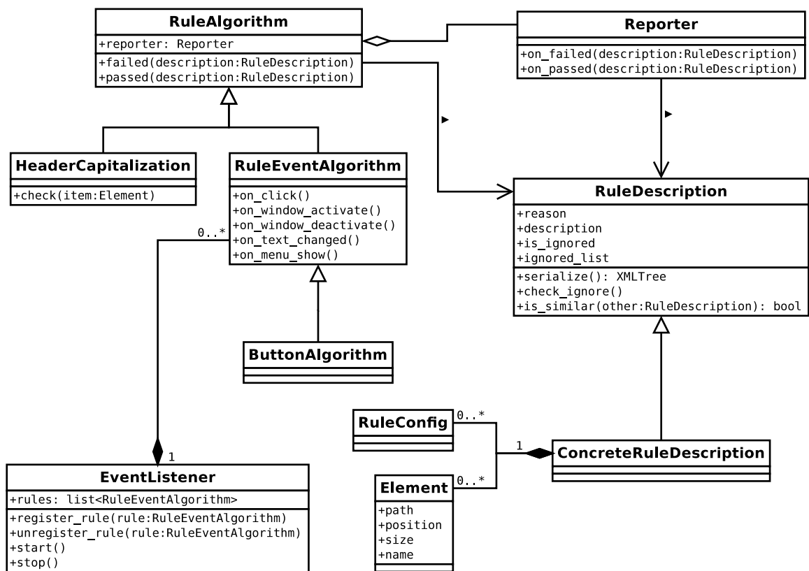
Obrázek 4.1: UML diagram tříd
