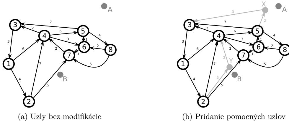
Obr. 4.11: Príklad grafu pre vyhľadávanie najkratšej cesty s uzlami
