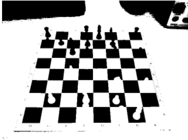
Obr 4.2 – aplikovanie prahovania
