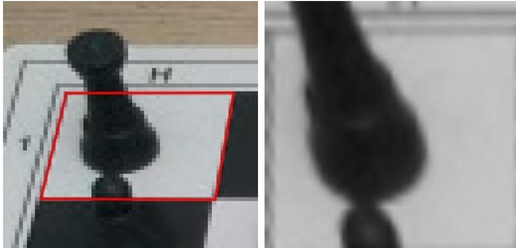
Obr 5.7 – perspektívna transformácia
