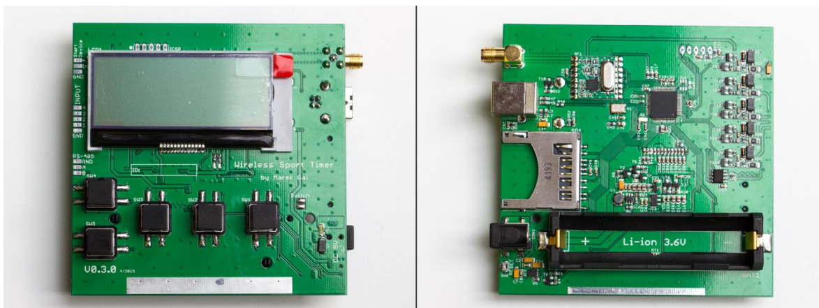
Obrázek 2-Deska primární jednotky
