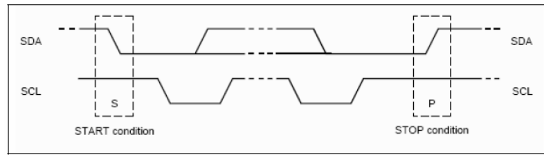
Obrázek 7-I2C zahájení a ukončení komunikace [8]
