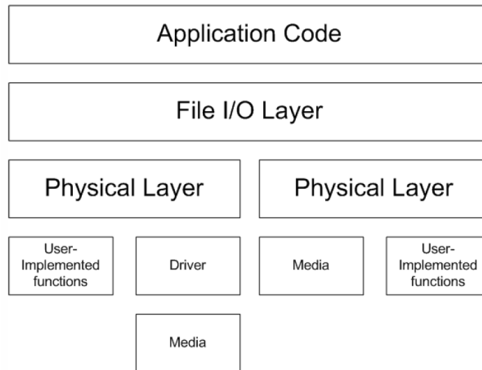
Obrázek 14-Struktura souborové knihovny
