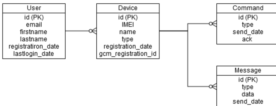
Obrázek 16 ER diagram
