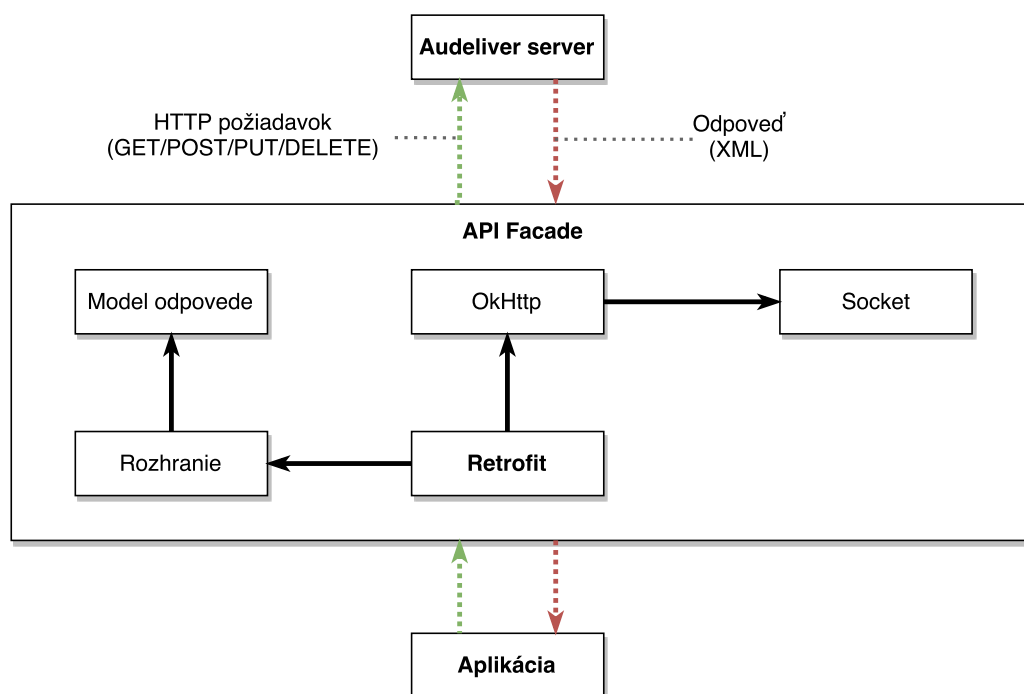
Obr. 5.2: Konceptuálny diagram implementácie komunikácie aplikácie so službou Audeliver. Plné čiary predstavujú závislosti medzi časťami aplikačného rozhrania. Prerušované čiary znázorňujú komunikáciu a jej smer.
