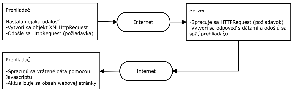
Obr. 4.2: Neblokujúca komunikácia so serverom pomocou AJAXu
