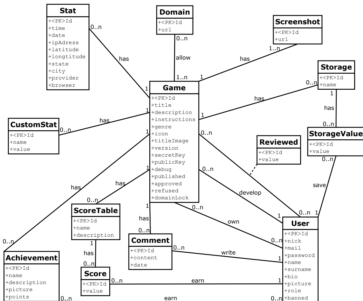
Obr. 3.12: Návrh databáze ako ER diagram
