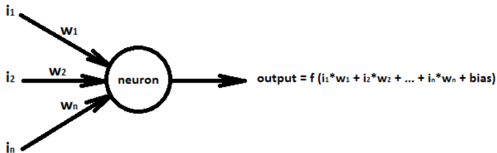
Obrázek 2: Perceptron
