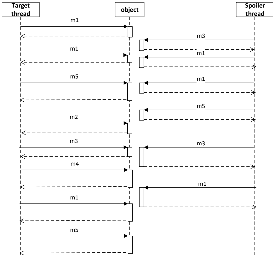
Obrázek B.16: Diagram testu 16.
