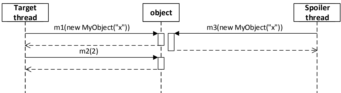
Obrázek B.35: Diagram testu 35.
