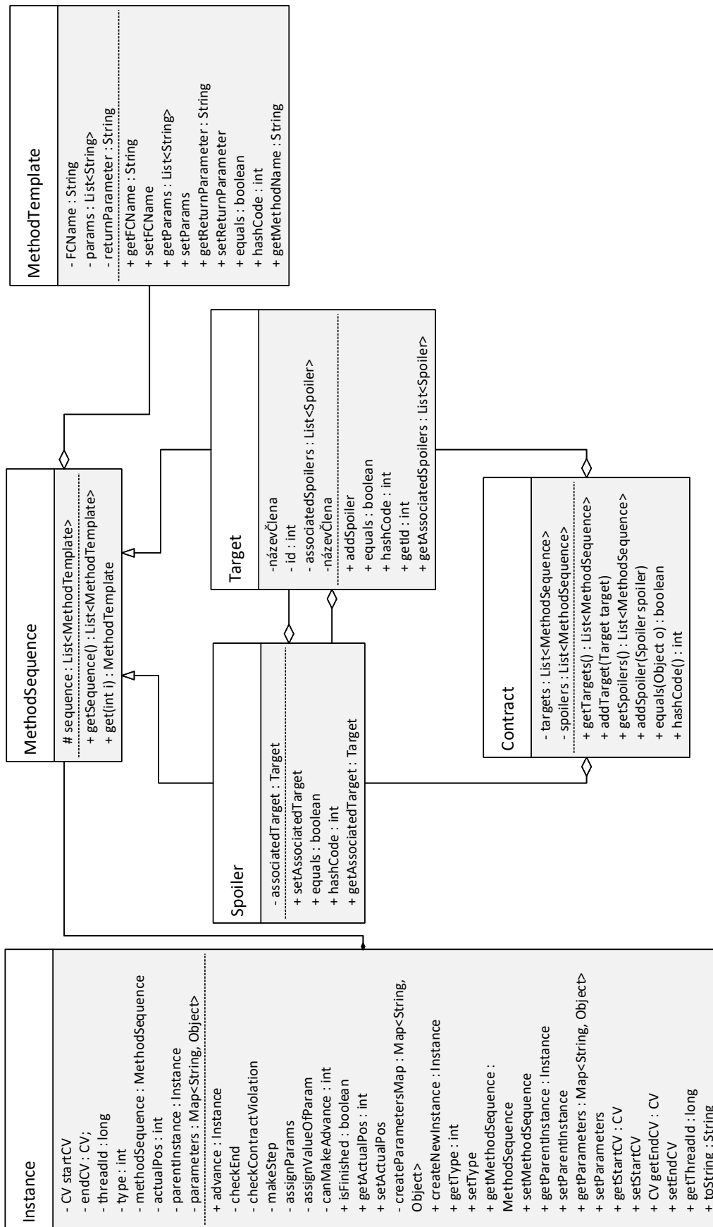
Obrázek 4.2: Diagram zobrazující třídy Target , Spoiler , Instance a jim přidružené třídy.
