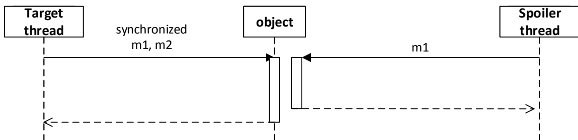
Obrázek B.2: Diagram testu 2.
