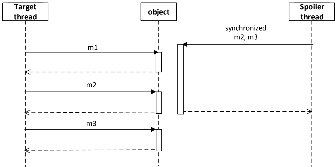
Obrázek B.10: Diagram testu 10.
