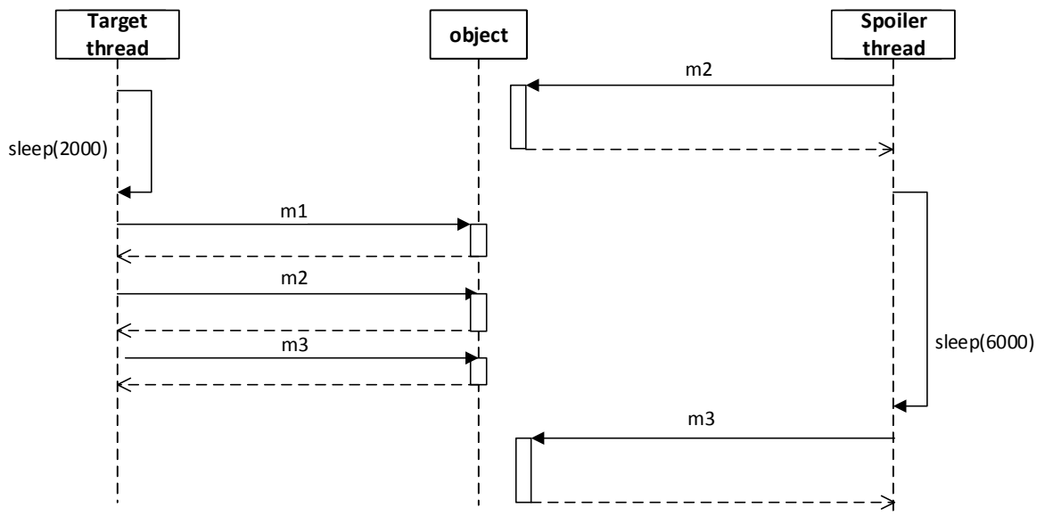
Obrázek B.11: Diagram testu 11.
