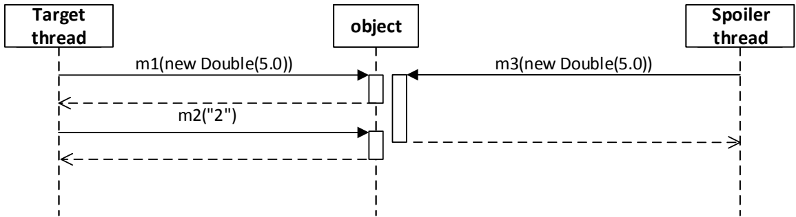
Obrázek B.34: Diagram testu 34.
