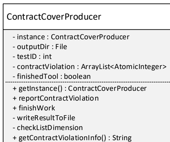
Obrázek 4.5: Diagram zobrazující třídu ContractCoverProducer.
