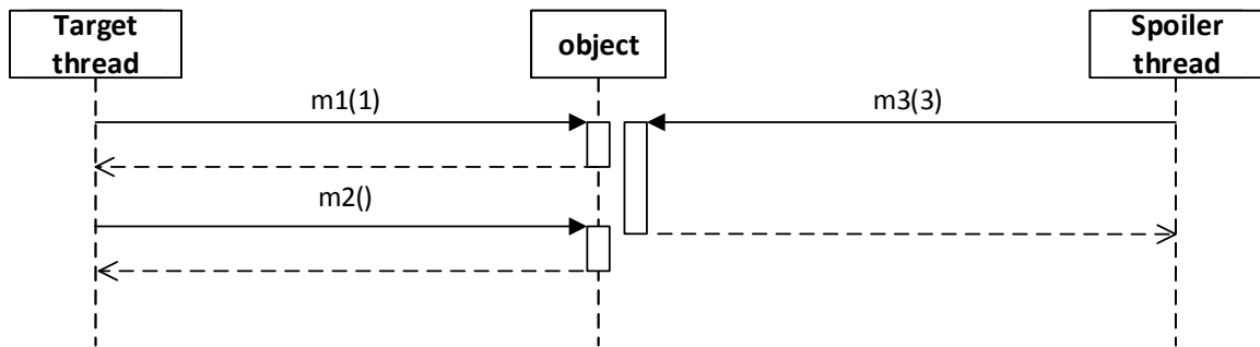
Obrázek B.30: Diagram testu 30.
