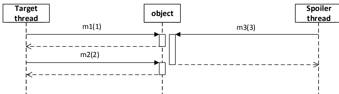
Obrázek B.29: Diagram testu 29.
