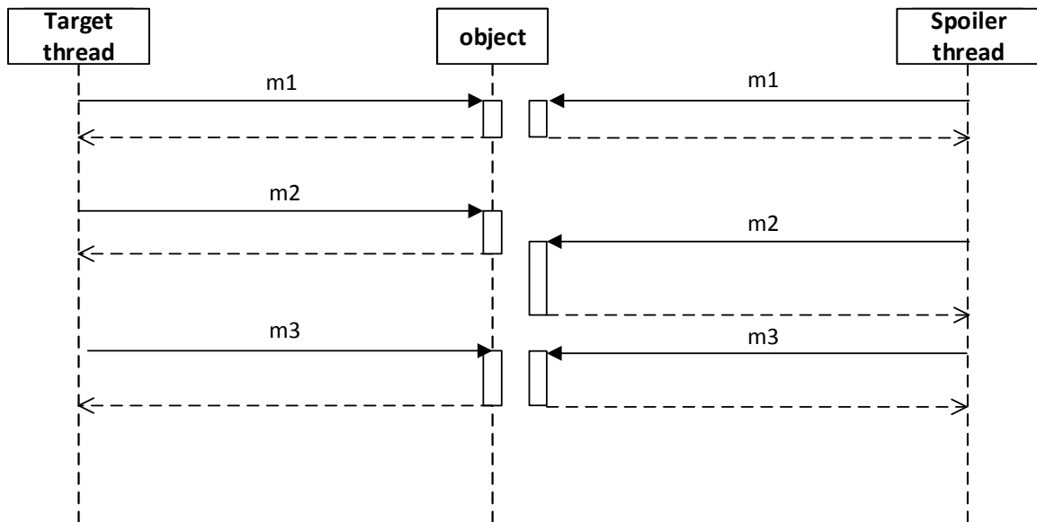
Obrázek B.24: Diagram testu 24.
