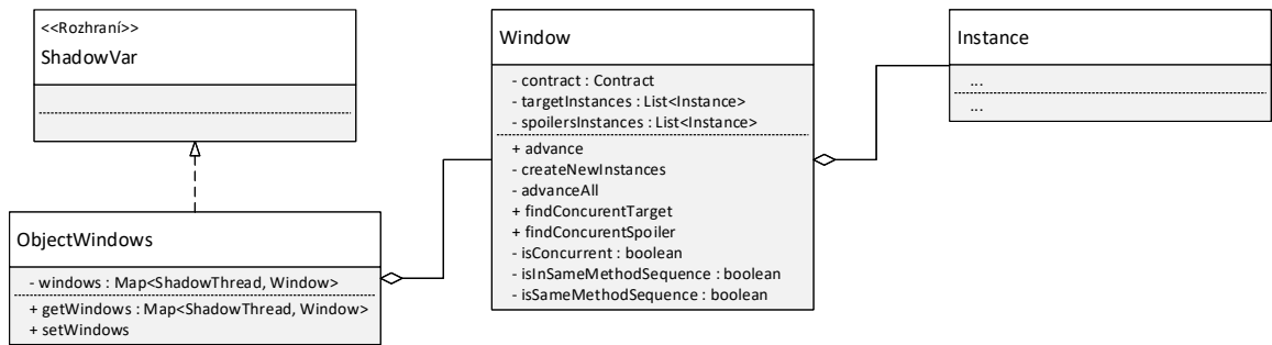
Obrázek 4.3: Diagram zobrazující třídu ObjectWindows a jí přidružené třídy.
