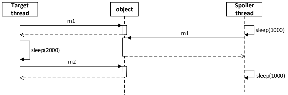
Obrázek B.5: Diagram testu 5.
