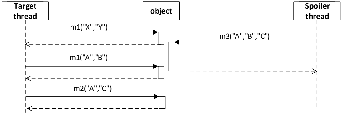
Obrázek B.40: Diagram testu 40.
