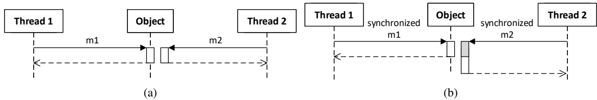
Obrázek 6.2: (a) Souběžné a (b) výlučné volání metod stejného objektu.
