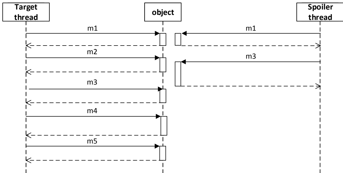
Obrázek B.19: Diagram testu 19.
