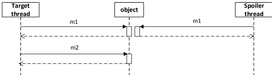
Obrázek B.4: Diagram testu 4.
