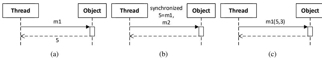
Obrázek 6.3: (a), (b) Volání metod s návratovou hodnotou a (c) s parametry.
