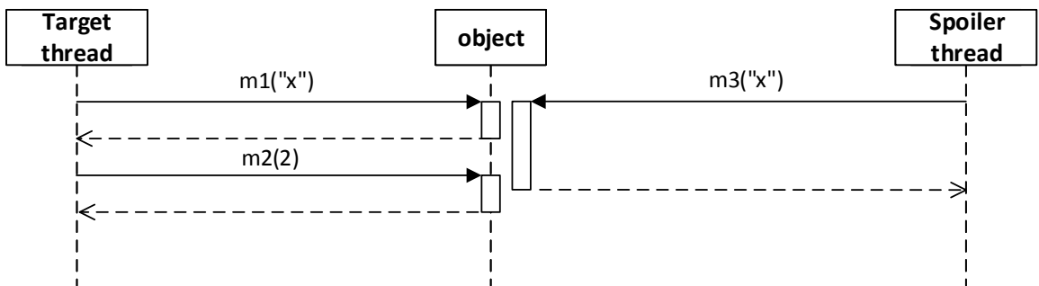
Obrázek B.33: Diagram testu 33.
