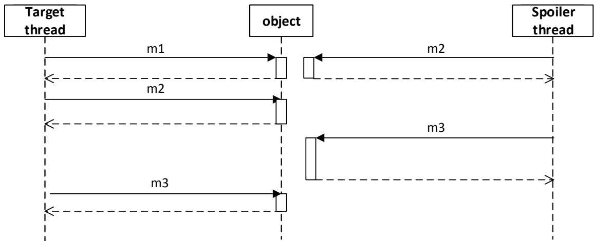
Obrázek B.8: Diagram testu 8.
