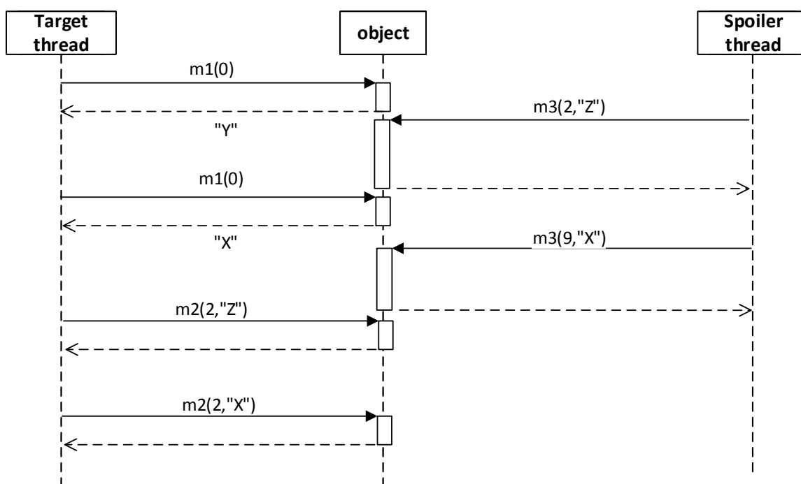
Obrázek B.46: Diagram testu 46.
