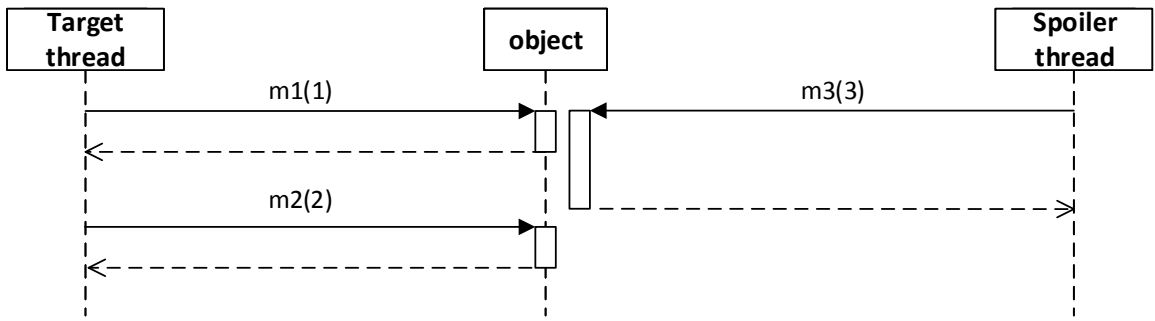
Obrázek B.36: Diagram testu 36.
