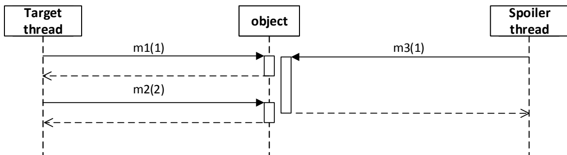
Obrázek B.31: Diagram testu 31.
