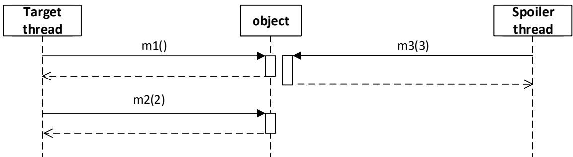
Obrázek B.37: Diagram testu 37.
