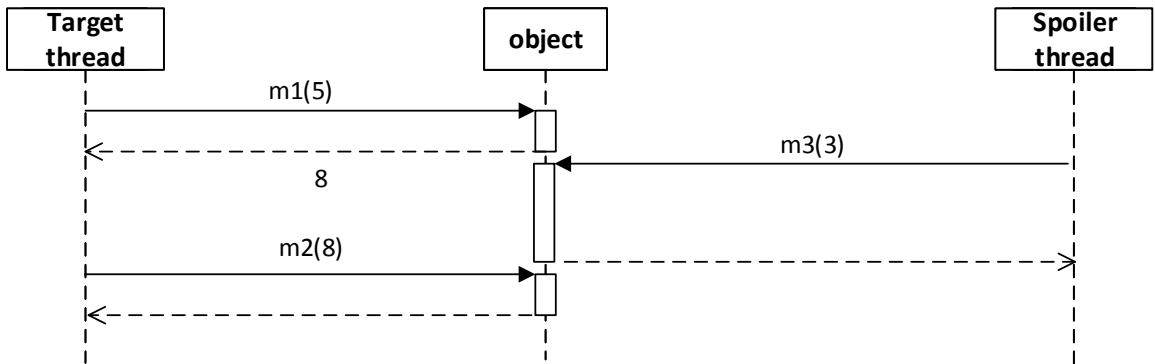
Obrázek B.42: Diagram testu 42.
