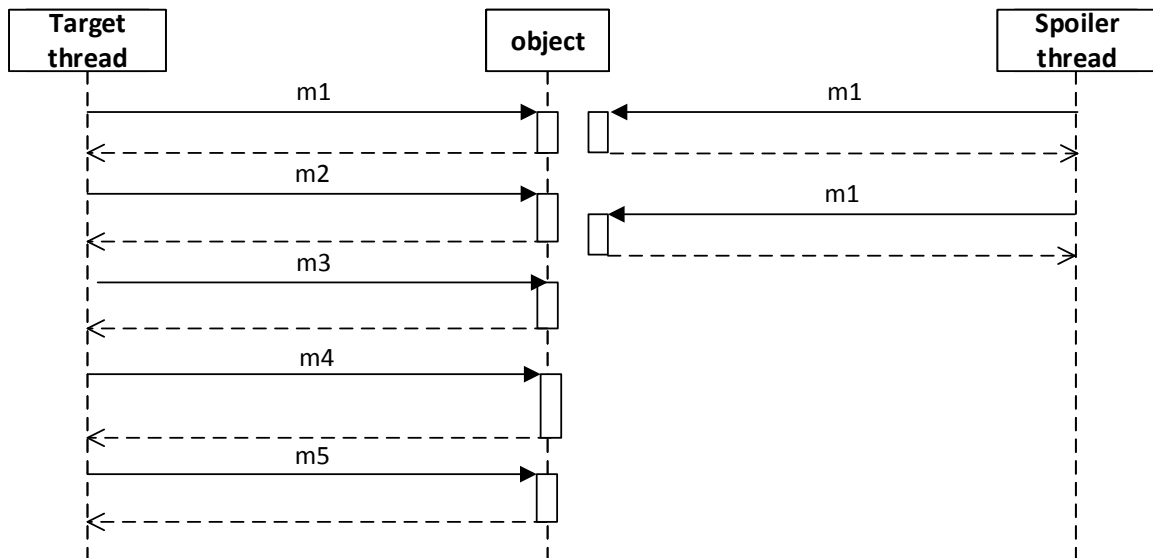
Obrázek B.20: Diagram testu 20.
