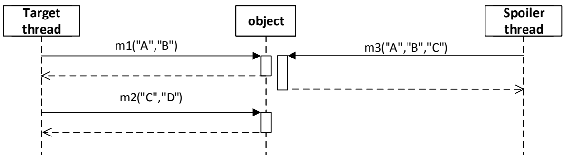
Obrázek B.39: Diagram testu 39.
