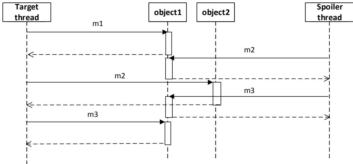
Obrázek B.23: Diagram testu 23.
