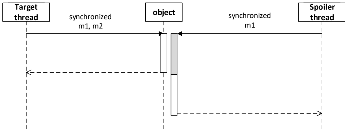
Obrázek B.1: Diagram testu 1.
