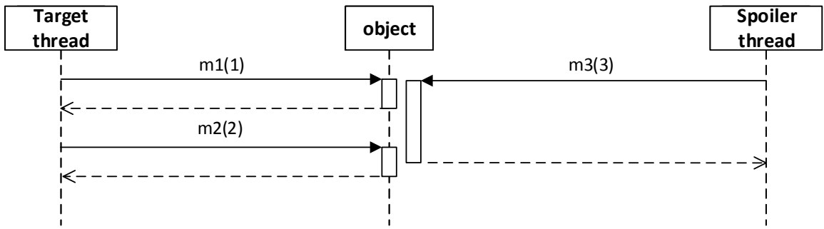
Obrázek B.32: Diagram testu 32.
