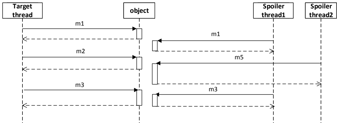
Obrázek B.26: Diagram testu 26.
