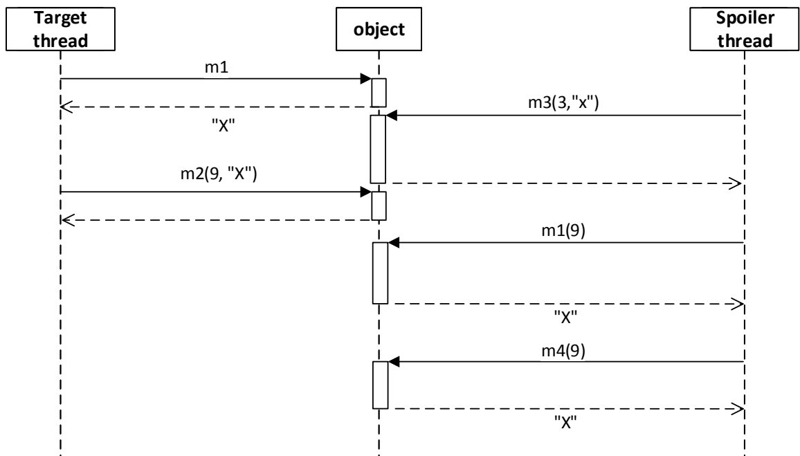
Obrázek B.45: Diagram testu 45.
