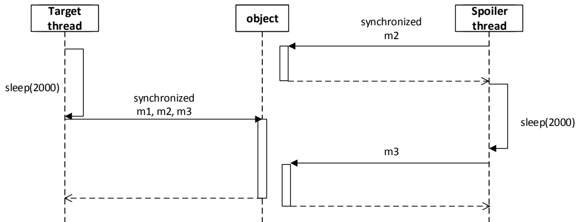
Obrázek B.12: Diagram testu 12.
