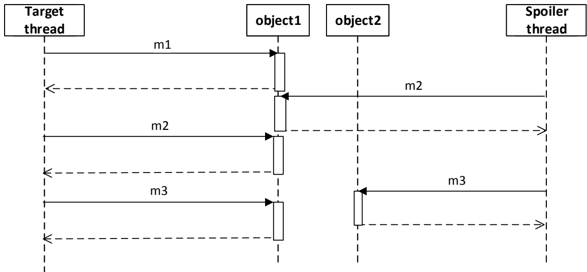
Obrázek B.22: Diagram testu 22.
