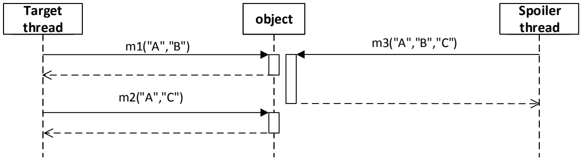
Obrázek B.38: Diagram testu 38.
