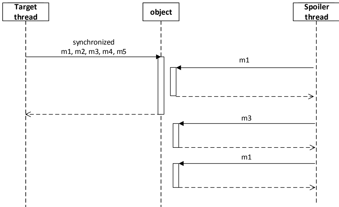
Obrázek B.14: Diagram testu 14.
