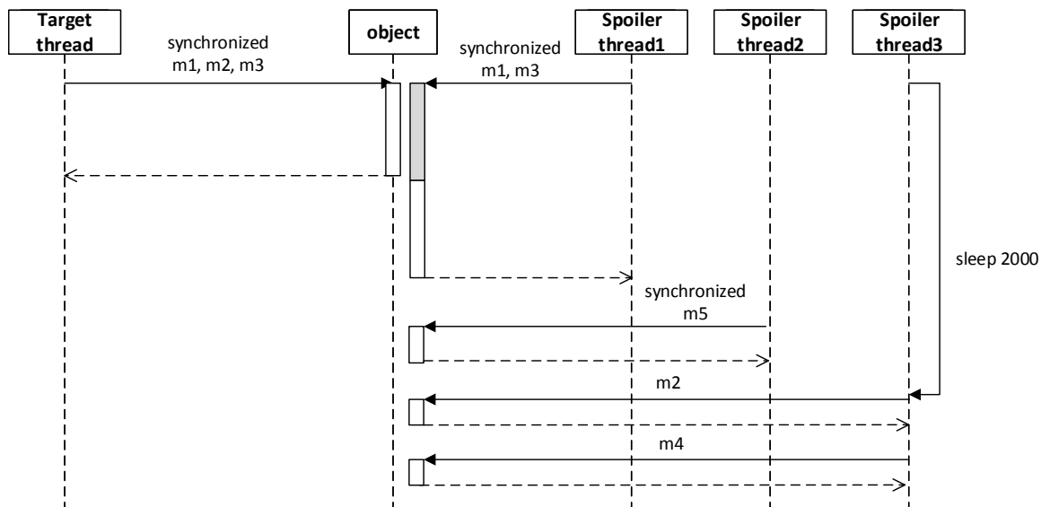
Obrázek B.28: Diagram testu 28.
