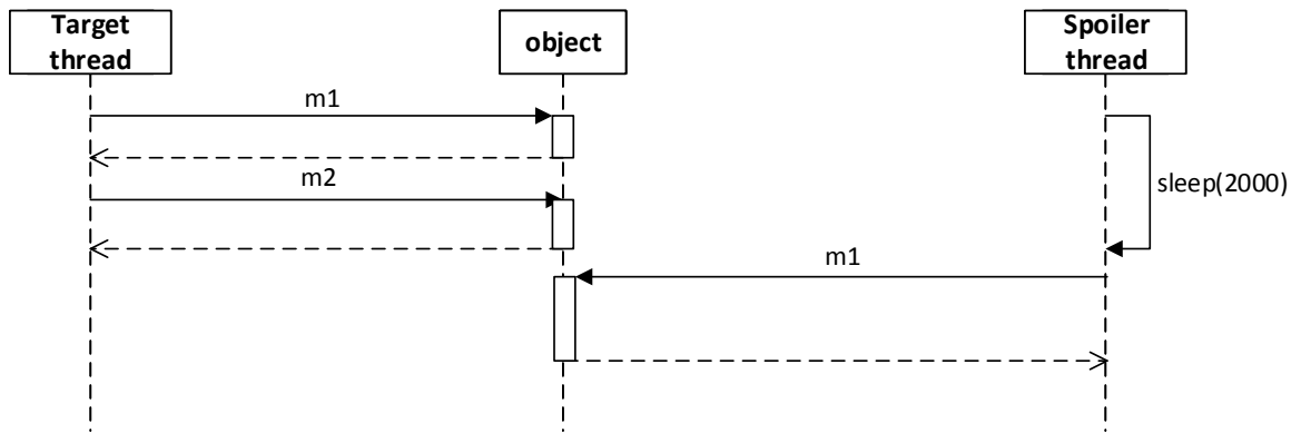
Obrázek B.7: Diagram testu 7.
