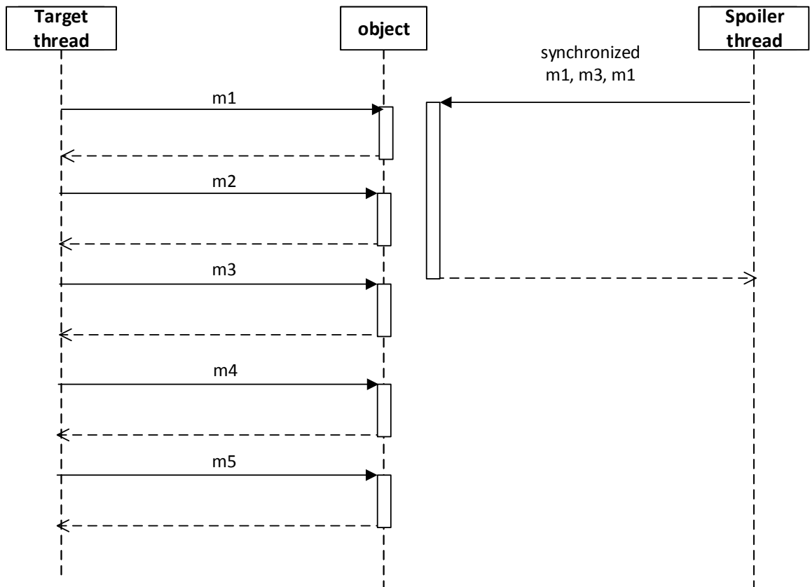
Obrázek B.15: Diagram testu 15.
