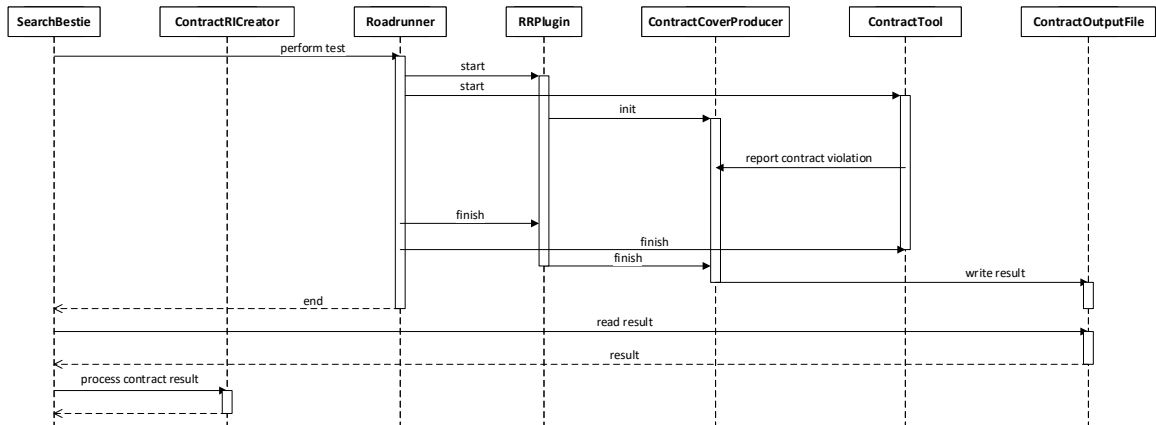
Obrázek 4.1: Konkrétní komunikace mezi komponentami dynamického analyzátoru kontraktů a SearchBestie.
