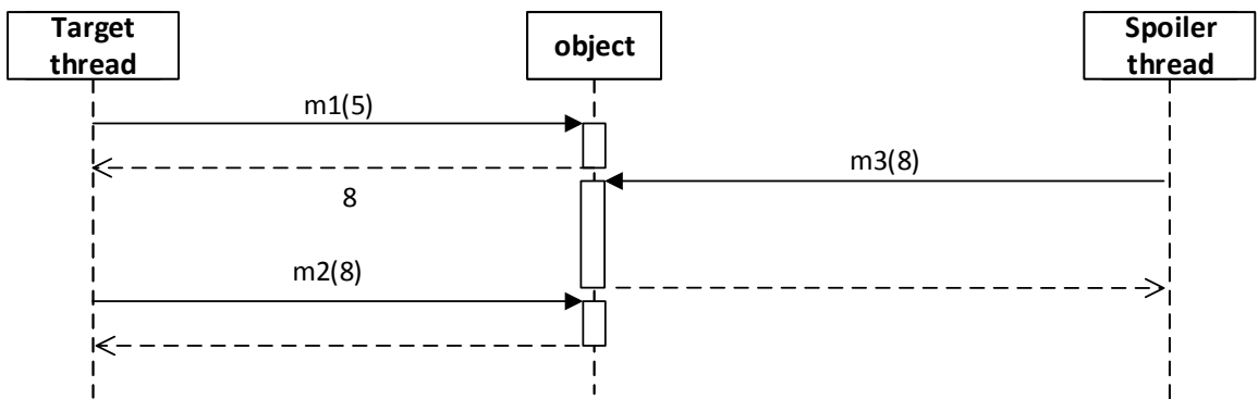
Obrázek B.41: Diagram testu 41.
