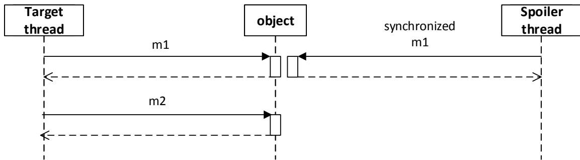
Obrázek B.3: Diagram testu 3.
