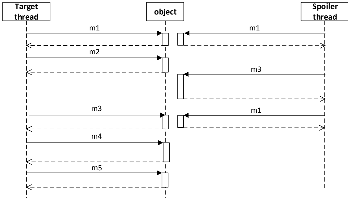
Obrázek B.13: Diagram testu 13.
