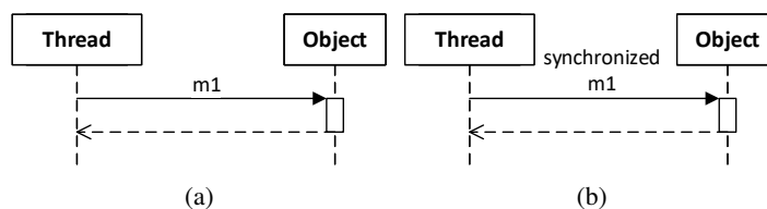
Obrázek 6.1: Volání metody s použitím (a) a bez použití (b) synchronizace.
