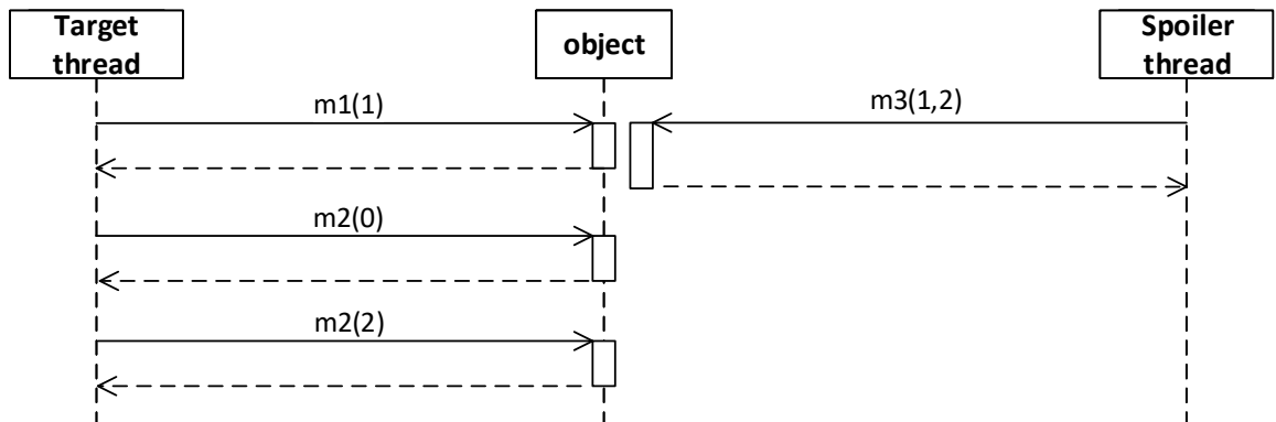
Obrázek 4.4: Příklad volání metod nad stejným objektem s různými parametry.
