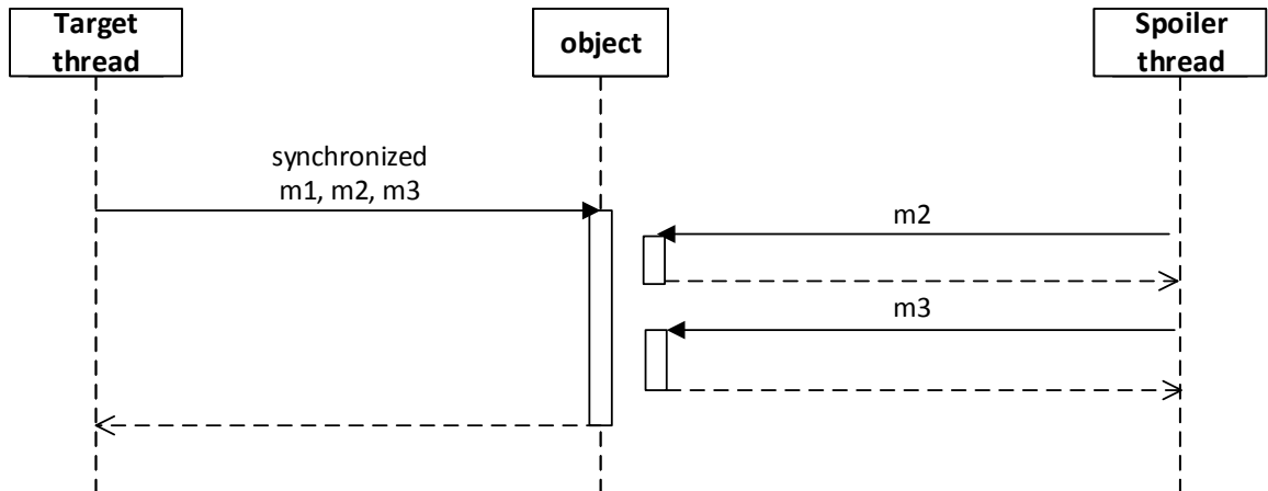
Obrázek B.9: Diagram testu 9.
