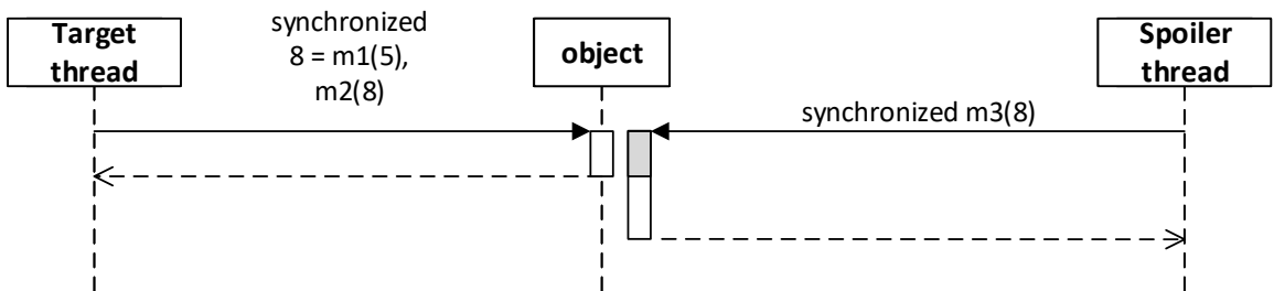
Obrázek B.43: Diagram testu 43.
