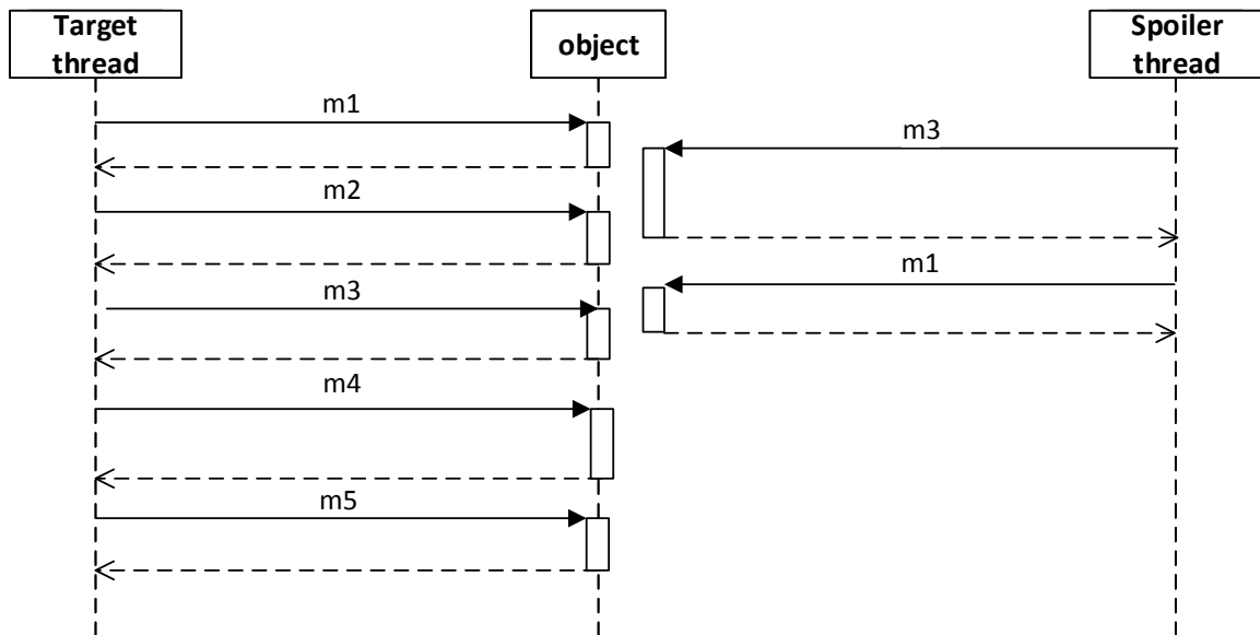
Obrázek B.18: Diagram testu 18.
