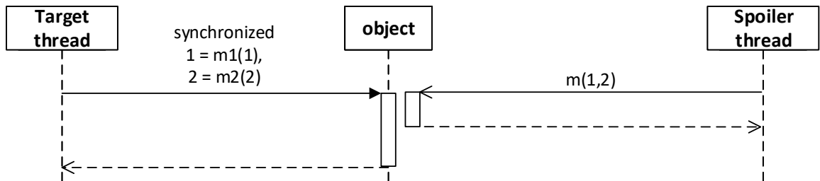
Obrázek B.44: Diagram testu 44.
