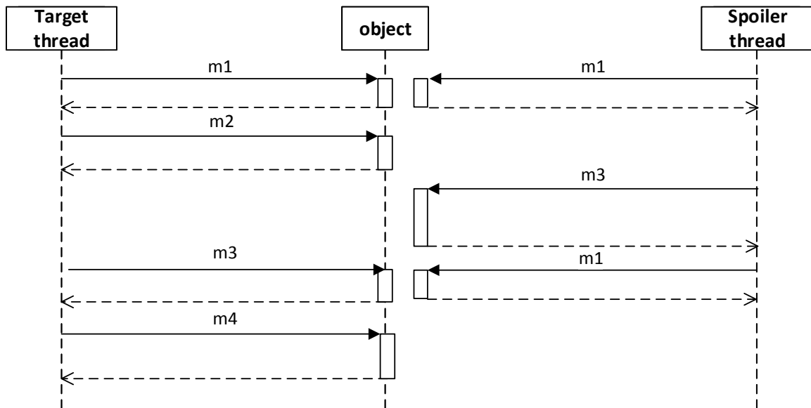
Obrázek B.17: Diagram testu 17.
