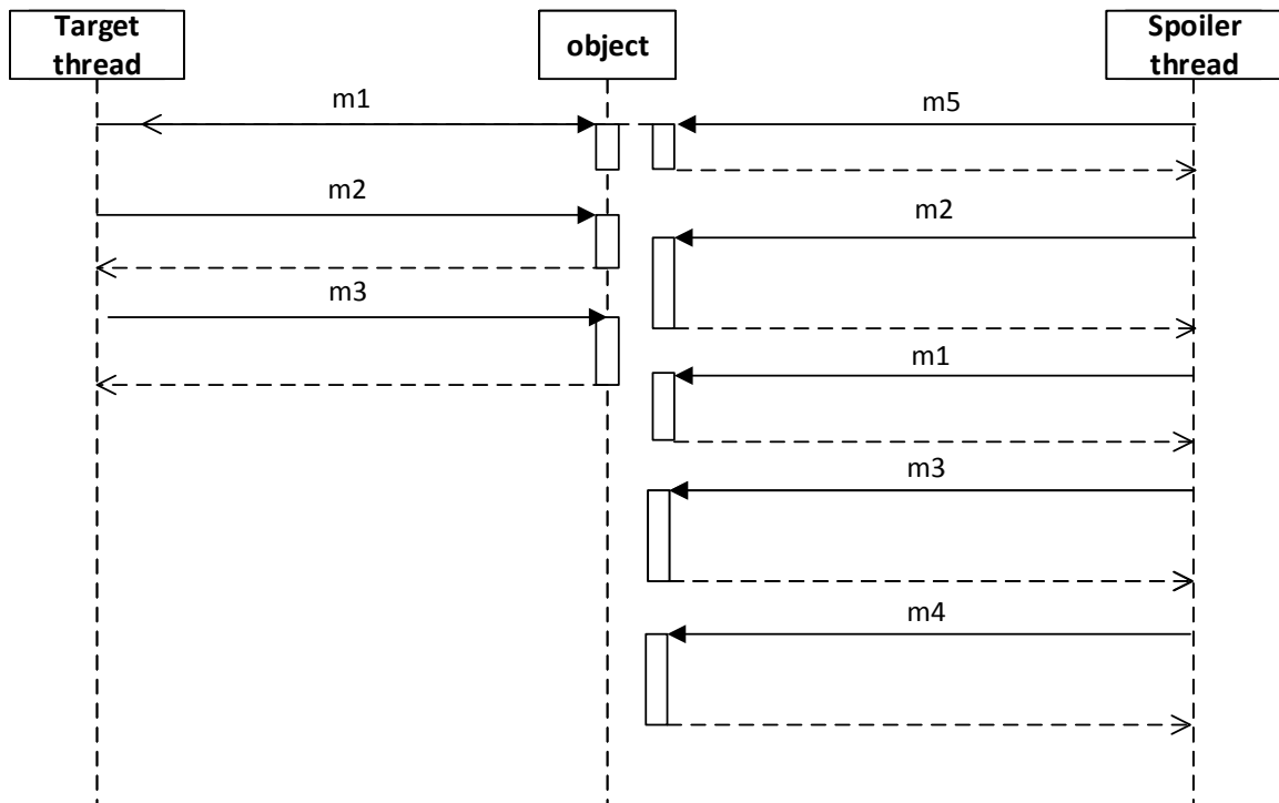
Obrázek B.25: Diagram testu 25.
