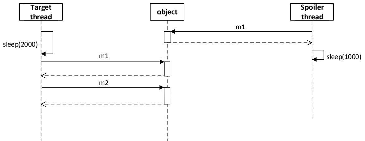
Obrázek B.6: Diagram testu 6.
