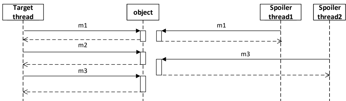
Obrázek B.27: Diagram testu 27.
