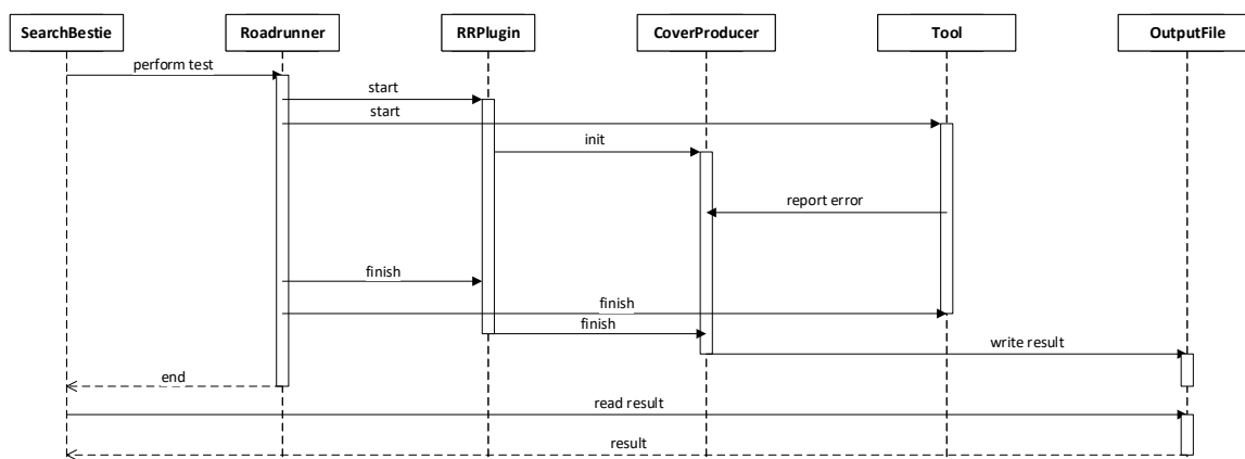
Obrázek 2.1: Komunikace v systému.
