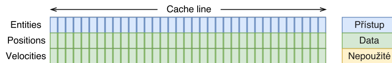
Obrázek 2.11: Využití procesorové vyrovnávací paměti při použití datově orientované kompozice.
