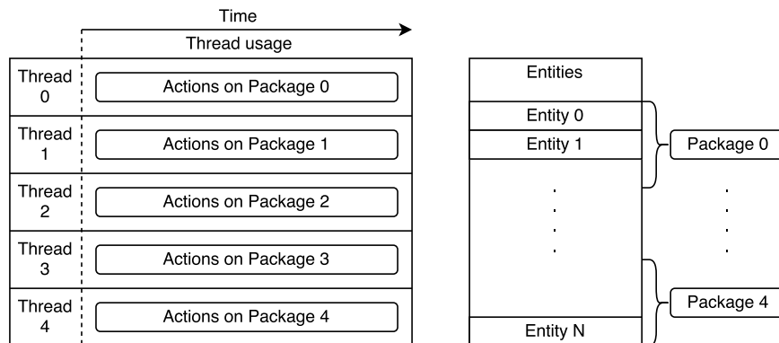
Obrázek 2.16: Paralelizmus uvnitř systémů je příkladem datového paralelizmu [9].
