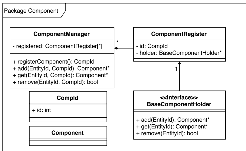
Obrázek 3.3: Diagram tříd podsystemu správy komponent .
