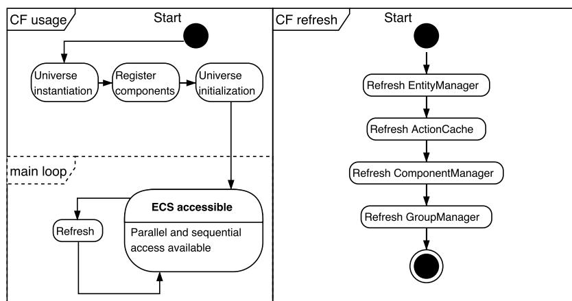
Obrázek 3.10: Diagram toku řízení entitního systému.
