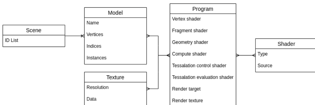
Obrázek 3.4: Diagram popisující jak vypadá scéna, která je výstupem knihovny. Zakončení čar symbolizuje vztah mezi prvky. Jednoduché značí 1:n, větvené m:n
