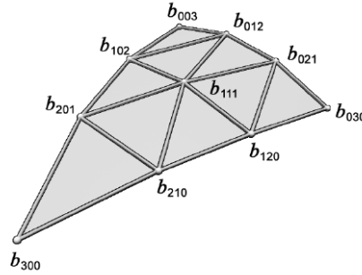
Obrázek 2.2: Ukázka rozdělení trojúhelníků pomocí techniky Curved PN triangles. 6
