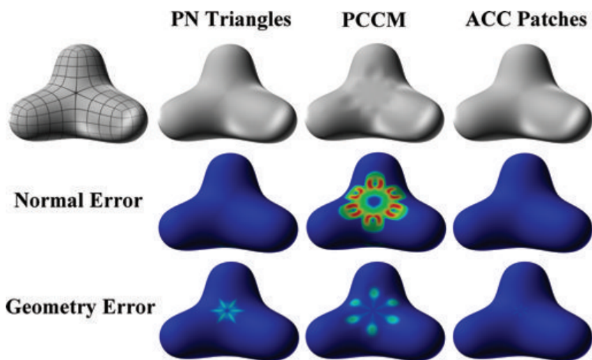
Obrázek 3.1: Porovnání metod zvyšování rozlišení geometrie. Každý z povrchů byl rozdělán dvakrát, každý jinou metodou. U PCCM vzniká relativně vysoká chyba normál, narozdíl od ostatních metod. 5
