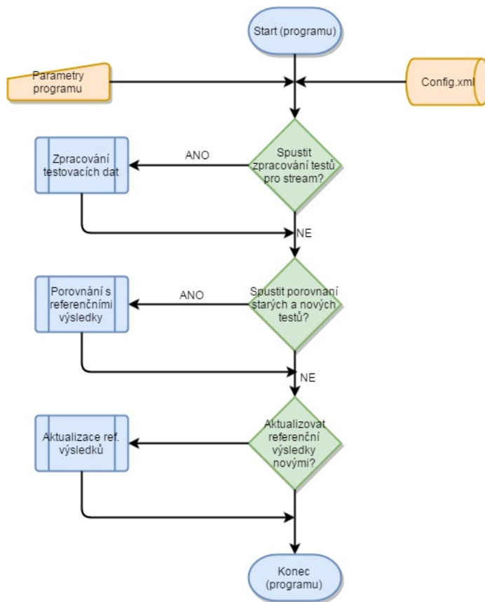
Obrázek 3.2: Tok programu
