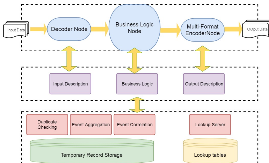
Obrázek 2.3: Prvky EventLinku
