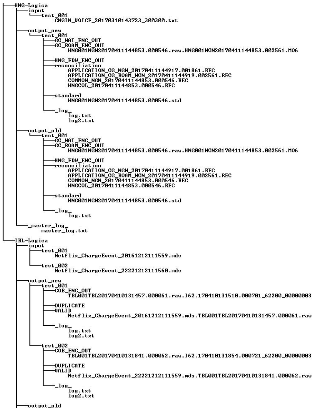
Obrázek 3.1: Struktura testovacích souborů
