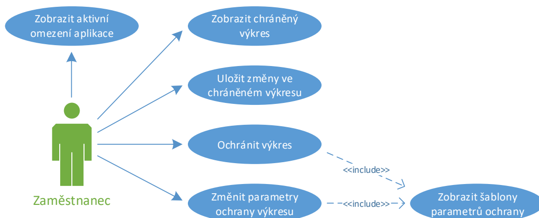
Obrázek 5.1: Diagram případů užití z pohledu zaměstnance.
