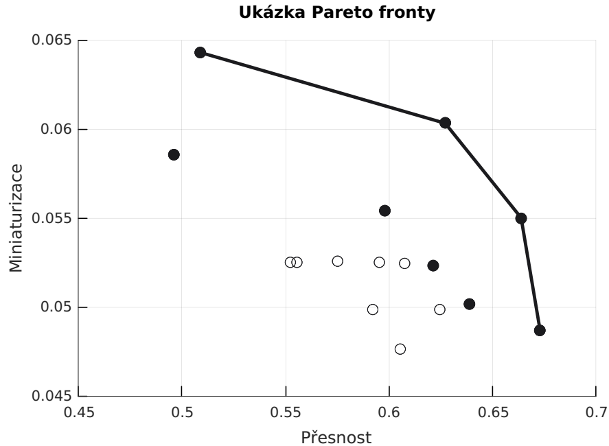
Obrázek 7.7: Ukázka vizualizace populace v jedné generaci. Plnou čarou jsou spojeni jedinci, kteří se nacházejí v Pareto frontě dané generace. Plnými kolečky jsou označeni jedinci, kteří byli vybráni do další generace. Prázdnými kolečky pak jedinci, kteří se do další generace nedostali.
