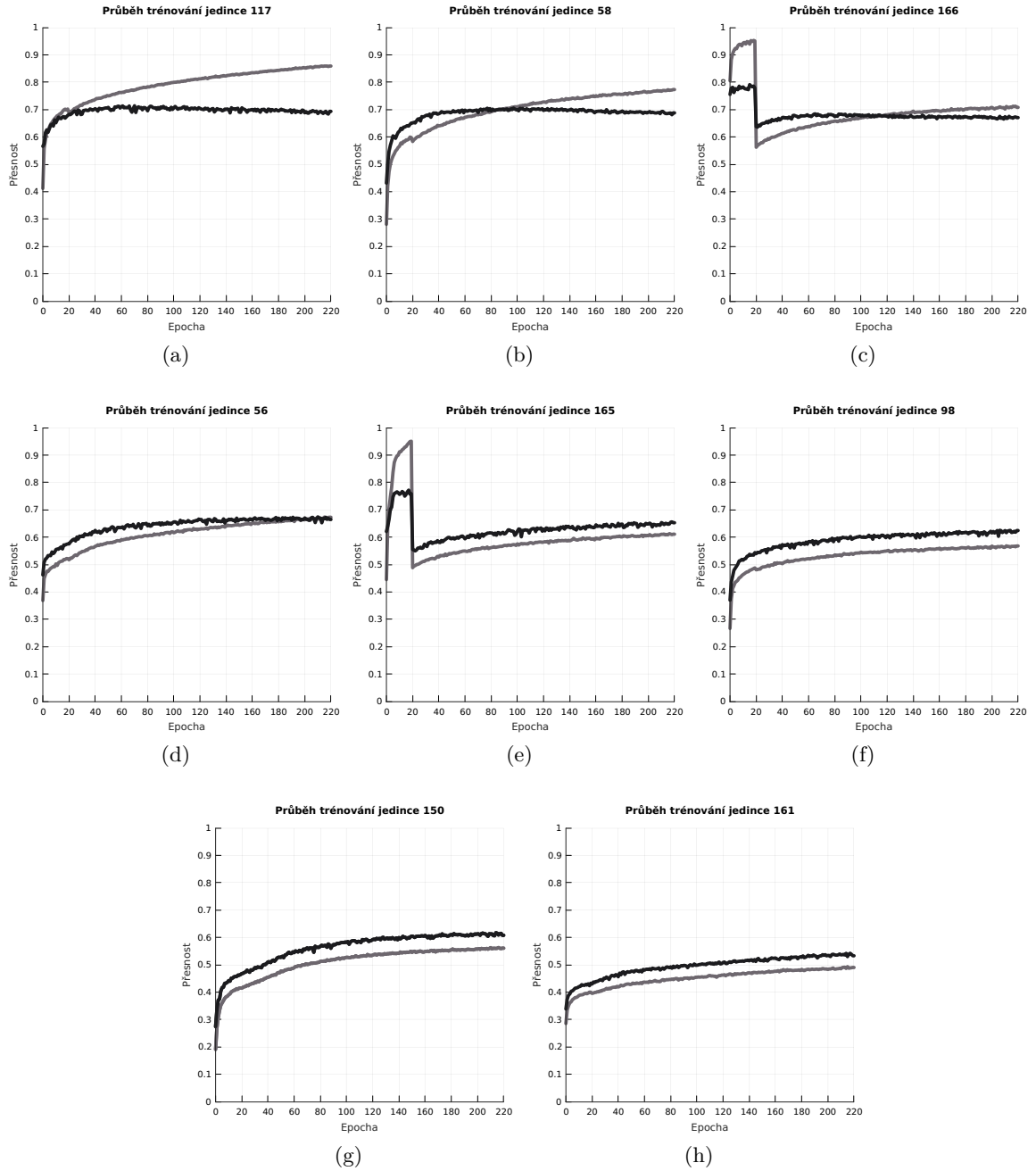
Obrázek A.2: Průběh učení nejlepších jedinců z experimentu, který využíval pouze jednoduché výpočetní uzly.
