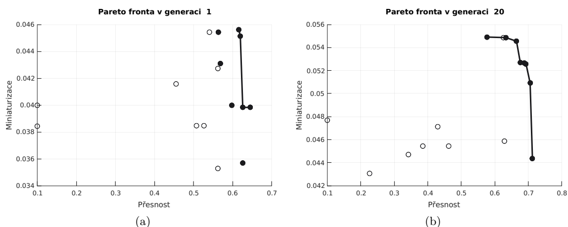
Obrázek B.1: Ukázka Pareto front ve vybraných generacích experimentu, který využíval reziduální výpočetní uzly.
