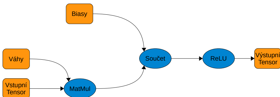
Obrázek 6.2: Příklad jednoduchého výpočetního grafu. Výstupní tenzory výpočetních uzlů MatMul a Součet zde nejsou naznačeny.
