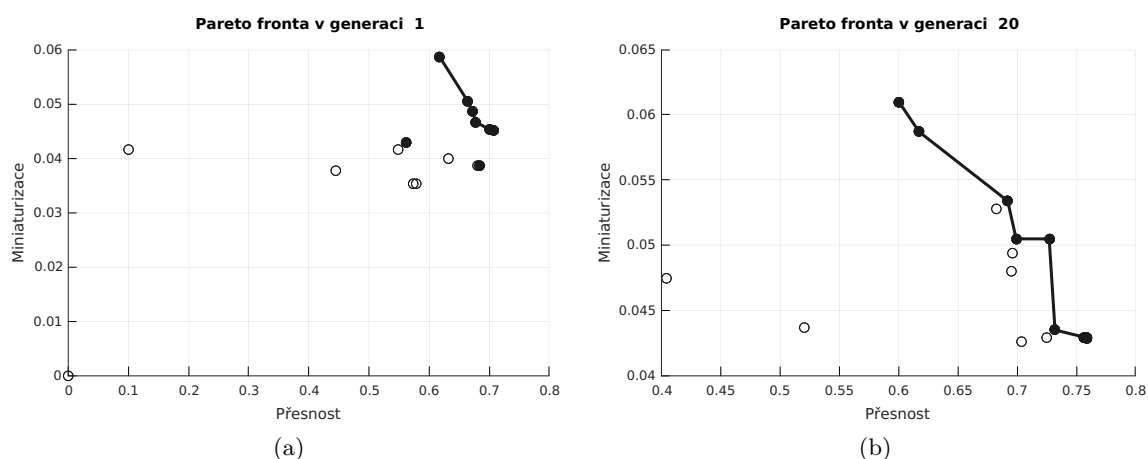
Obrázek C.1: Ukázka Pareto front ve vybraných generacích experimentu, který využíval inception výpočetní uzly.
