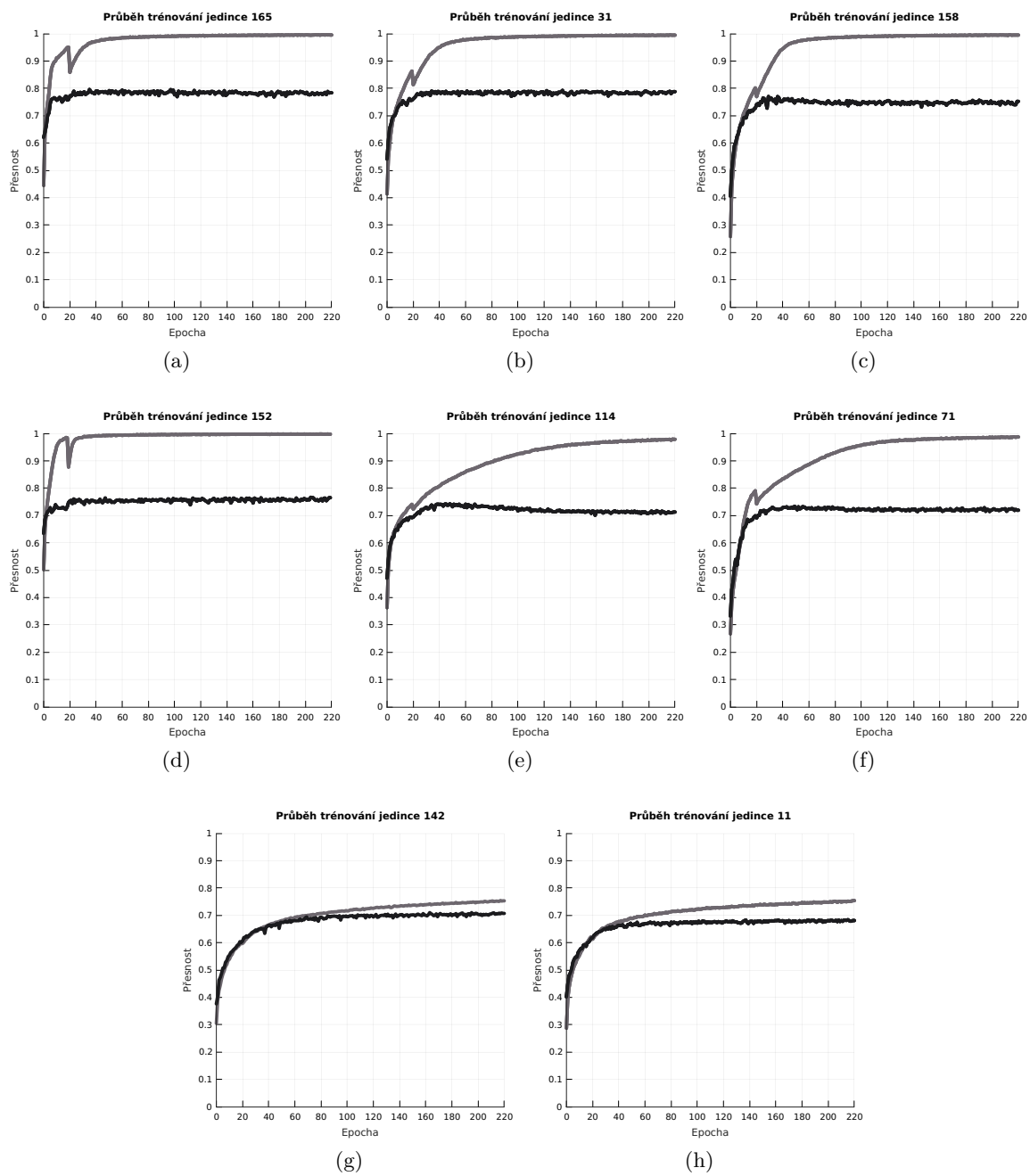
Obrázek C.2: Průběh učení nejlepších jedinců z experimentu, který využíval inception výpočetní uzly.
