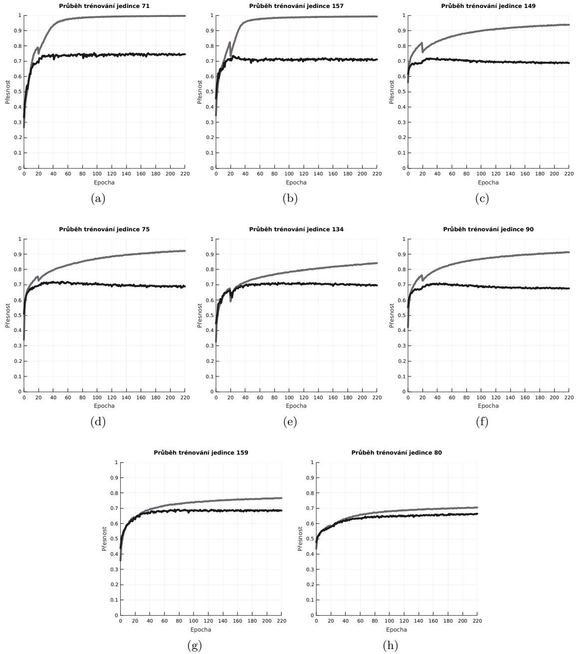
Obrázek B.2: Průběh učení nejlepších jedinců z experimentu, který využíval reziduální výpočetní uzly.
