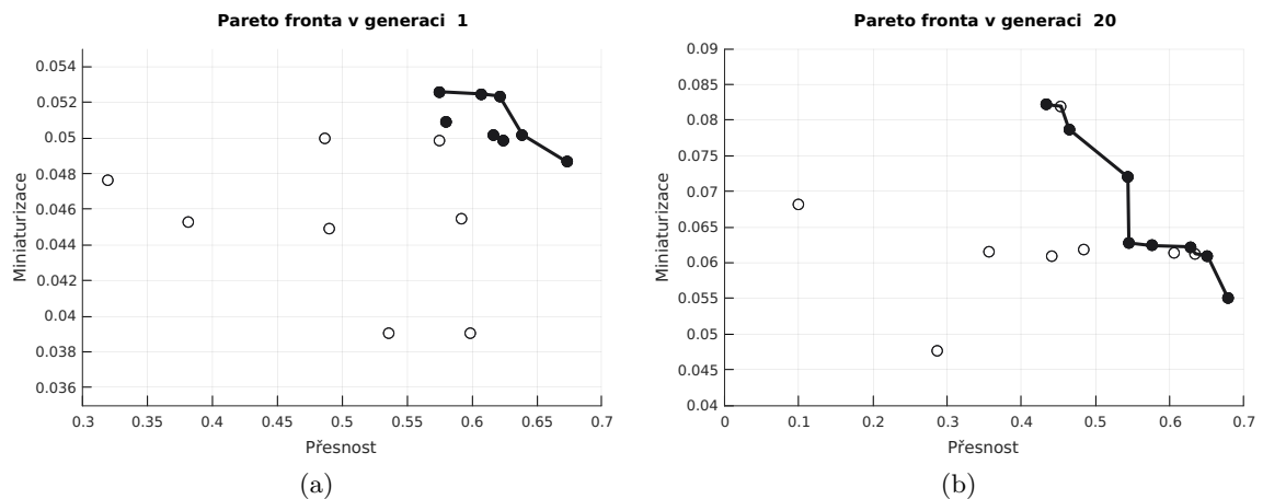
Obrázek A.1: Ukázka Pareto front ve vybraných generacích experimentu, který využíval pouze jednoduché výpočetní uzly.
