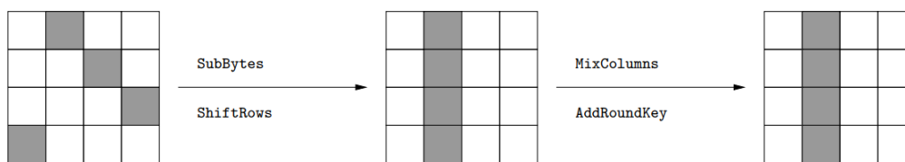
Obr. 3.5: Schématický náhľad na jedno kolo (iteráciu) algoritmu AES.
