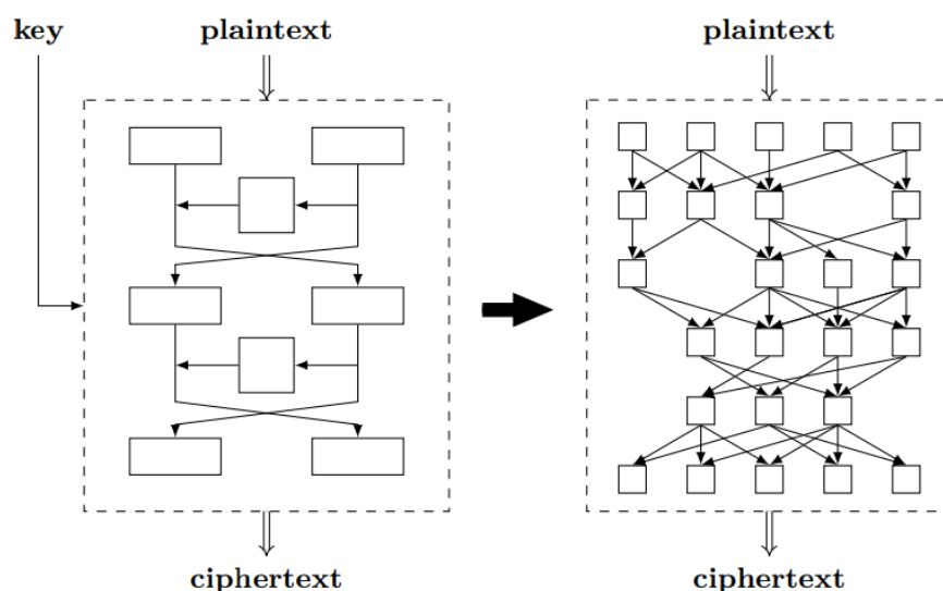
Obr. 3.4: V ľavo je algoritmus blokovej šifry založený na Feistelovej sieťovej štruktúre. V pravo, white-box implementácia tohoto šifrovacieho bloku kde je kľúč hard-kódovaný do algoritmu.
