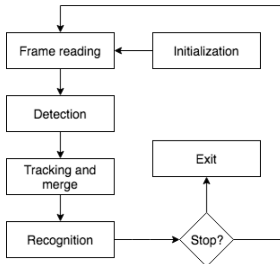
Obrázek 5.1: Algoritmus zpracování dat v uživatelské aplikaci.
