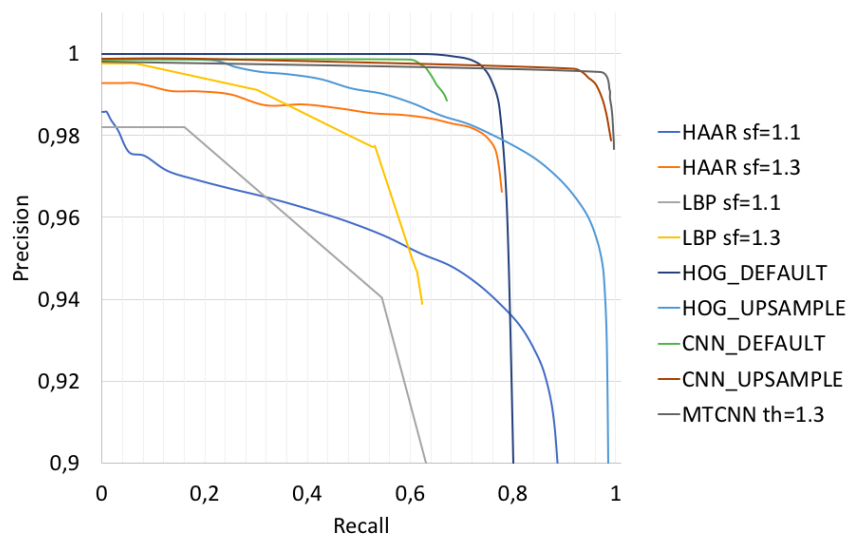
Obrázek 3.7: Porovnání precision - recall křivek všech testovaných metod.
