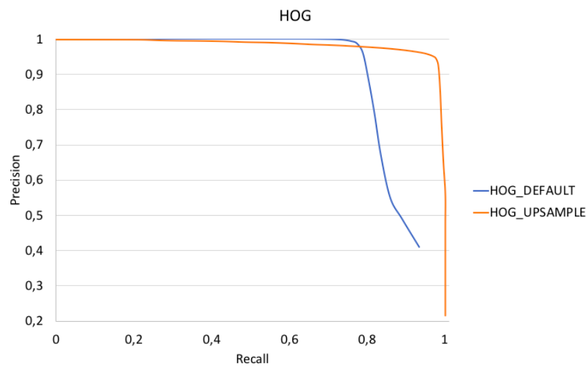
Obrázek 3.10: Precision - recall křivky pro různá nastavení parametru upsample metody HOG.
