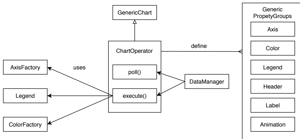
Obrázek 4.2: Blokové schéma reprezentující implementaci ChartOperator je libovolnou podtřídou generického operátoru. Informace pro povolení grafu (v metodě poll() ) a data pro tvorbu vizualizace jsou získávány ze třídy DataManager . V operátoru mohou být definovány skupiny vlastností, dle kterých se následně řídí v metodě execute tvorba vizualizace. V případě definice skupiny vlastností pro osy, legendu nebo barvu je vytvoření objektů nebo materiálů abstrahováno do tříd nacházejících se na schématu vlevo.
