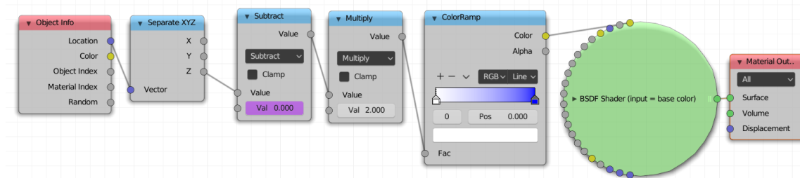
Obrázek 4.3: Node Shader pro obarvení grafů vytvořený pomocí kódu
