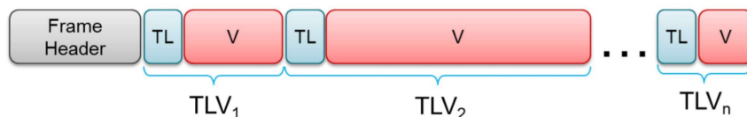
Obrázek 4.2: Rozdělení paketu radaru [3]
