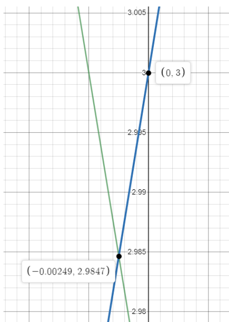
Obrázek 6.8: Na grafu je průsečík modré hyperboly, která má mikrofony přesně 1 metr vzdálené a zpoždění signálů odpovídá zdroji na pozici [0,3] , a zelené hyperboly, která má mikrofony vzdálené 1,01 metru a počítá se se vzdáleností 1 metr (chyba 1 cm).
