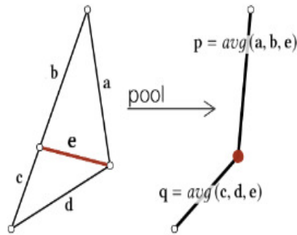
Obr. 3.9: Pooling operácia na štyroch susedných hranách. Výsledok sú dve nové hrany, ktoré sa spočítajú ako priemer vektoru rysov. Prevzaté z [16]
