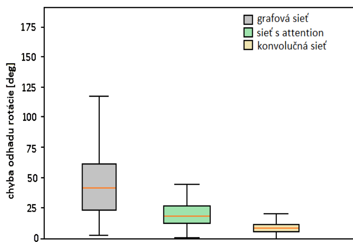
Obr. 5.7: Porovnanie výsledkov grafovej siete a baseline metódy.
