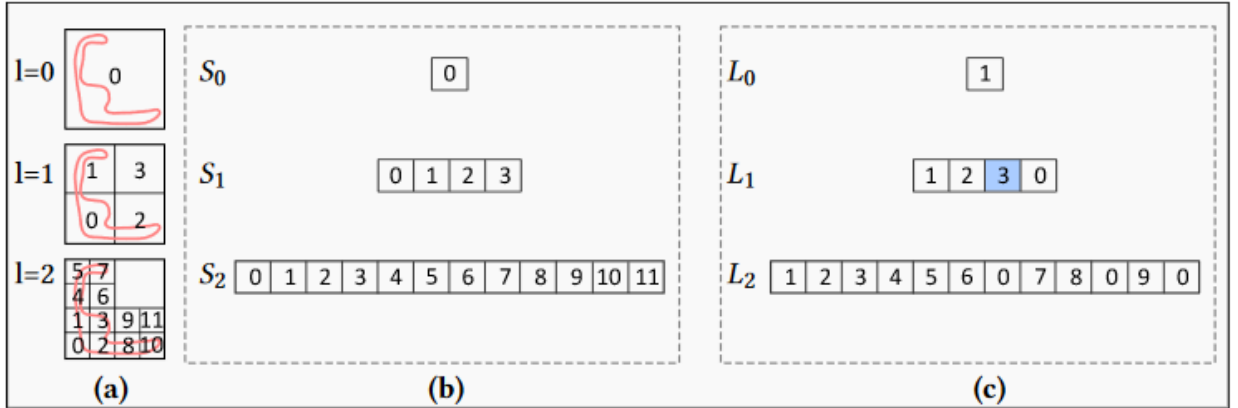
Obr. 3.10: Ukážka stromu. Obrázok a) ukazuje ako sa štvorec delí na menšie a menšie časti. Čísla reprezentujú shuffle key. Na obrázku b) sú už znázornené shuffle key v stromovej štruktúre. Na obráčku c) sa nachádzajú pridelené anotácie jednotlivým uzlom. Prevzaté z [32]
