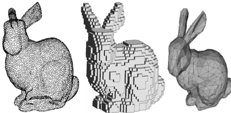
Obr. 2.2: Rôzne reprezentácie modelu. Vľavo sa nachádza point cloud, v strede je 3D mriežka a vpravo polygóniálny model. Prevzaté z [17].
