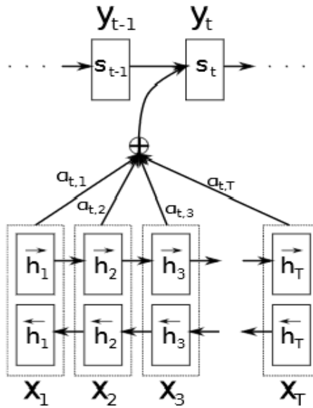
Obr. 3.15: Attention mechanizmus v encoder-dekocer sieti. Enkóder tu predstavujú spodné vrstvy h_1 až h_T . Dekóder zase vrstvy s_{t-1} a s_t . Kontextový vektor pre jeden výstup y_t sa počíta zo všetkých vrstiev enkóderu h_1 až h_T . Prevzaté z [8].
