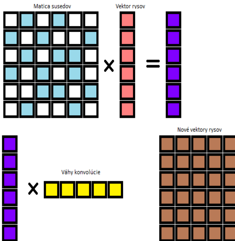
Obr. 3.12: Jednoduchý príklad ilustrujúci spôsob fungovania konvolučnej vrstvy v grafových sieťach.
