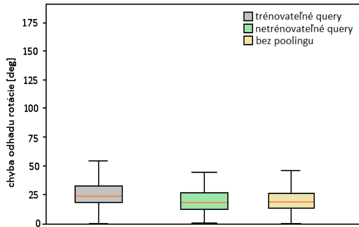
Obr. 5.5: Porovnanie experimentov pre sieť s attention. Graf vľavo patrí experimentu s trénovateľnými query vektormi, prostredný experimentu s netrénovateľnými query a pravý graf patrí experimentu bez pooling.
