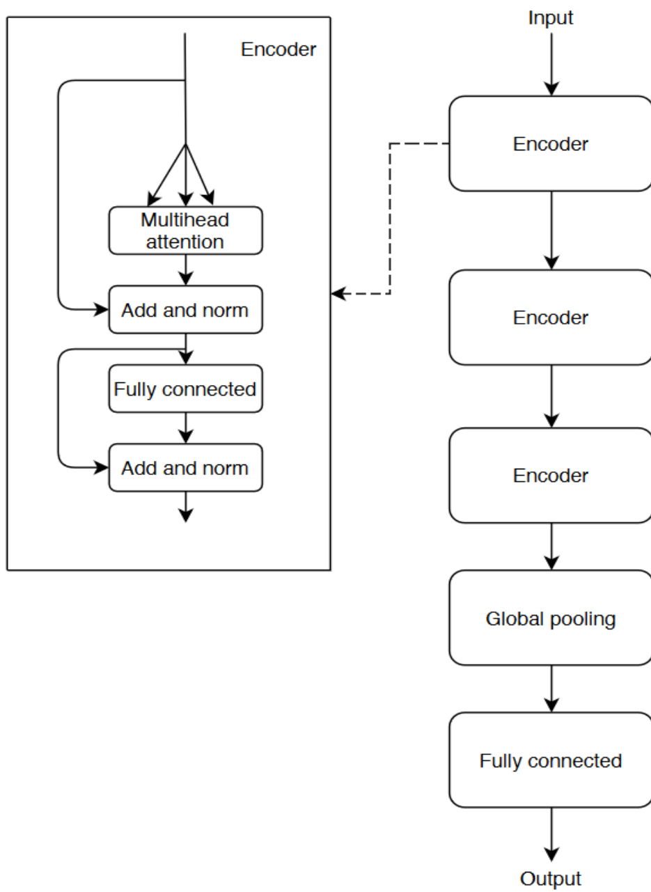
Obr. 4.11: Architektúra s attention mechanizmom bez pooling.
