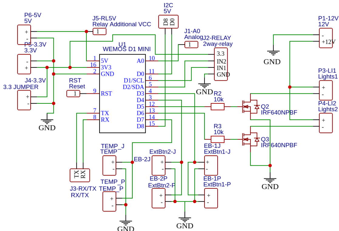
Obrázek B.1: Návrh schématu centrálního zařízení
