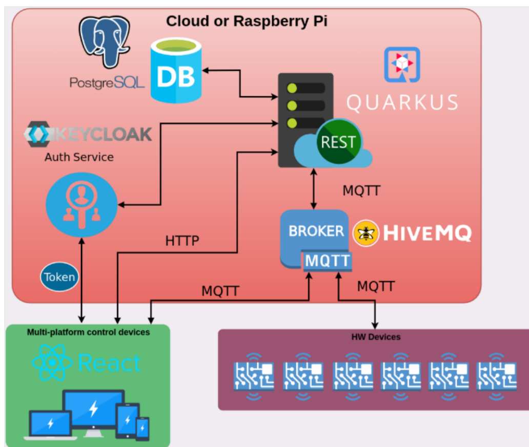
Obrázek 4.1: Použité služby v architektuře
