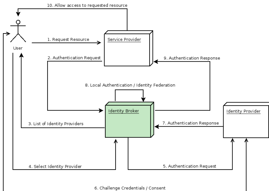
Obrázek 4.12: Autentizační tok KeyCloak . Převzato z [11].
