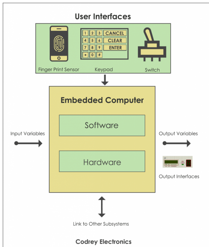
Obrázek 2.1: Koncept vestavěného systému. Převzato z [21].
