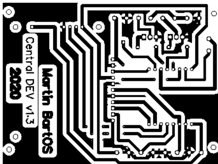
Obrázek B.2: Návrh DPS pro centrální zařízení
