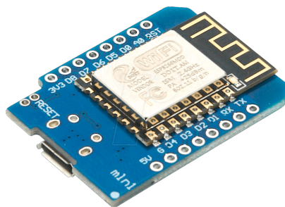
Obrázek 5.3: Modul Wemos D1 mini . Převzato z [17].
