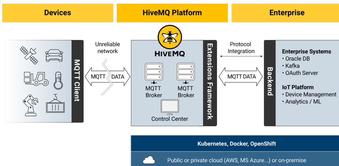
Obrázek 4.13: Enterprise architektura MQTT. Převzato z [5].
