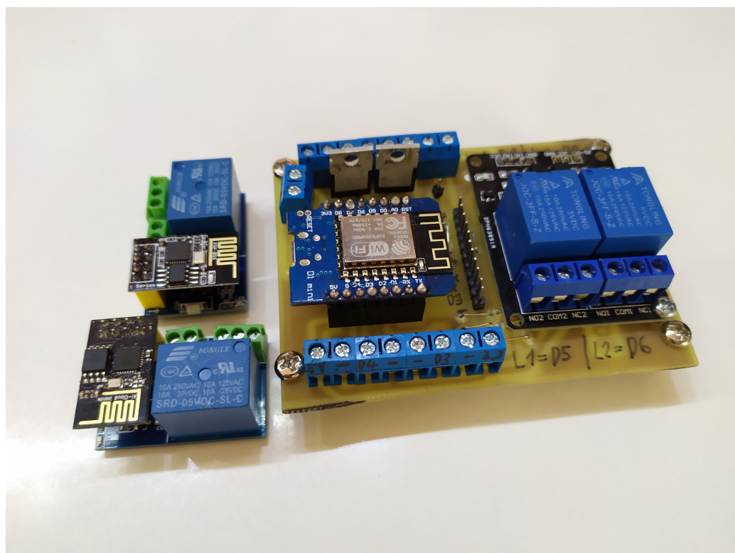
Obrázek B.3: Vyrobené centrální zařízení a 2 relé moduly s mikrokontrolérem ESP-01 .
