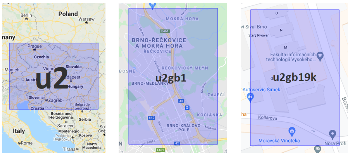
Obrázek 2.3: Zvyšování úrovně přesnosti kódování pomocí metody Geohash.
