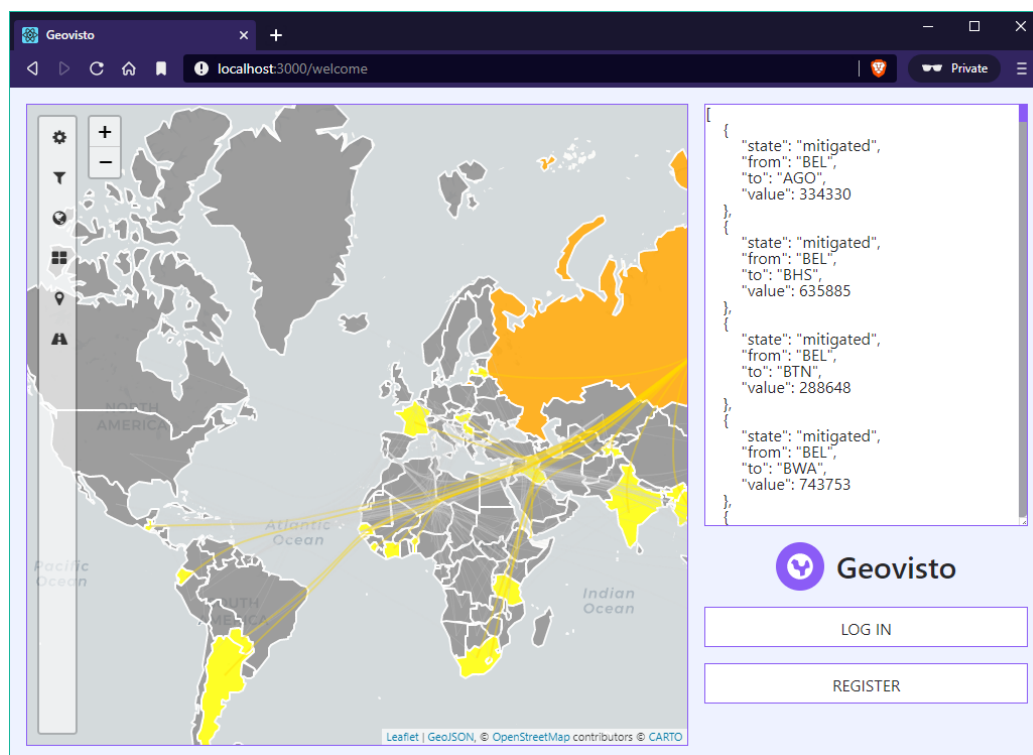
Obrázek A.1: Úvodní obrazovka obsahující oblast s komponentou pro vizualizaci a oblast představující zdroj dat. Uživatel může vyzkoušet funkcionalitu ještě před registrací do systému.
