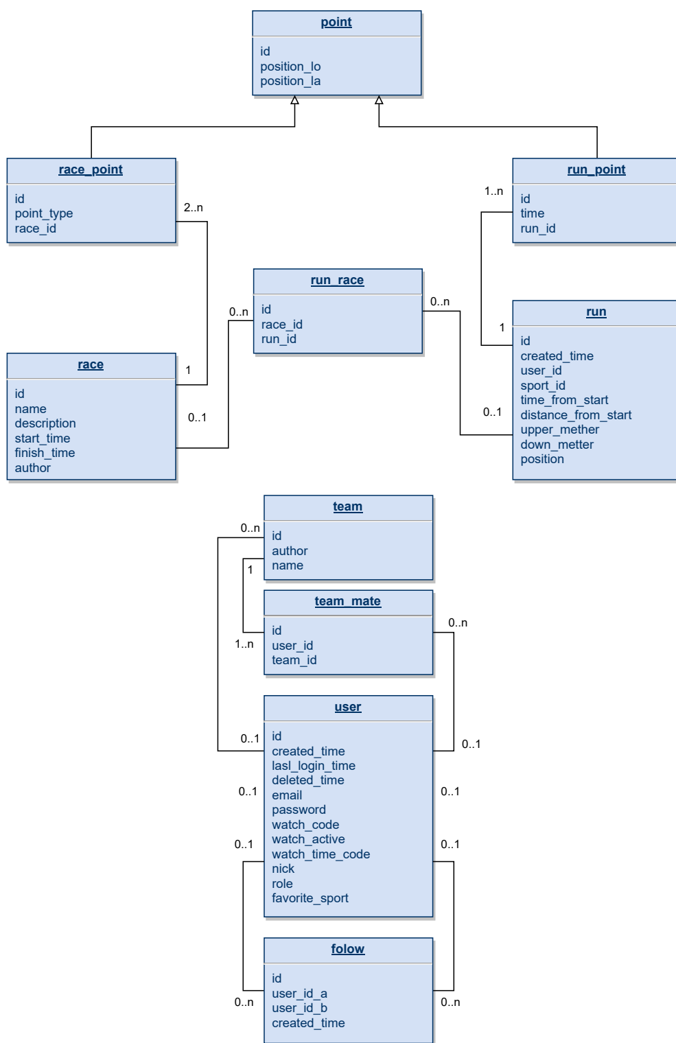
Obrázek 5.15: ER diagram databáze navržený pro moduly aplikačního serveru. Na horním obrázku databáze pro ukládání dat o závodě. V dolní části obrázku databáze pro ukládání uživatele.
