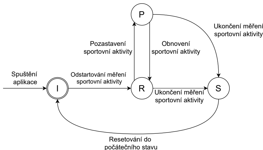
Obrázek 6.1: Diagram stavů, ve kterých se může aplikace nacházet. Přejchod mezi stavy je realizovaný interakcí s uživatelem.
