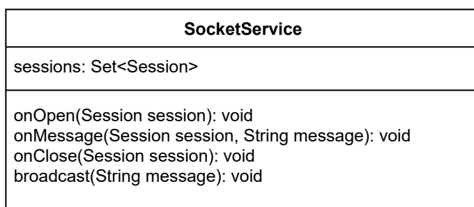
Obrázek 6.11: Schéma třídy SocketService s metodami pro zahájení komunikace, komunikaci, ukončení komunikace a pro hromadné odesílání zpráv.
