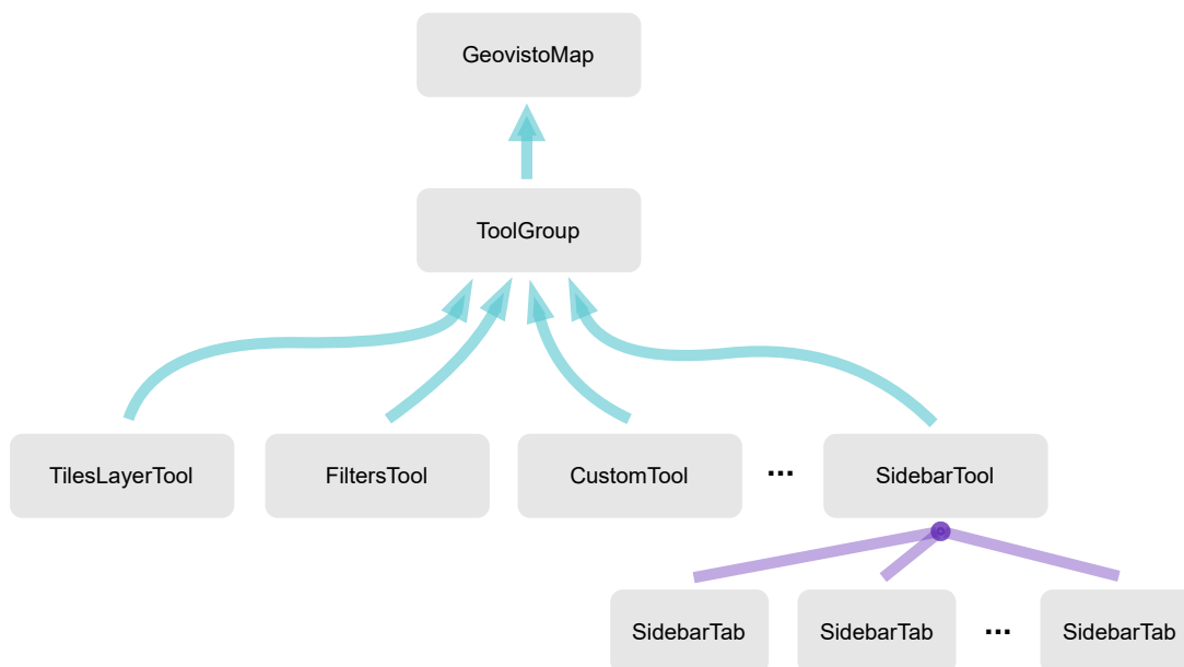
Obrázek 6.2: Tok dat při inicializaci nástrojů a vytváření tématické mapy
