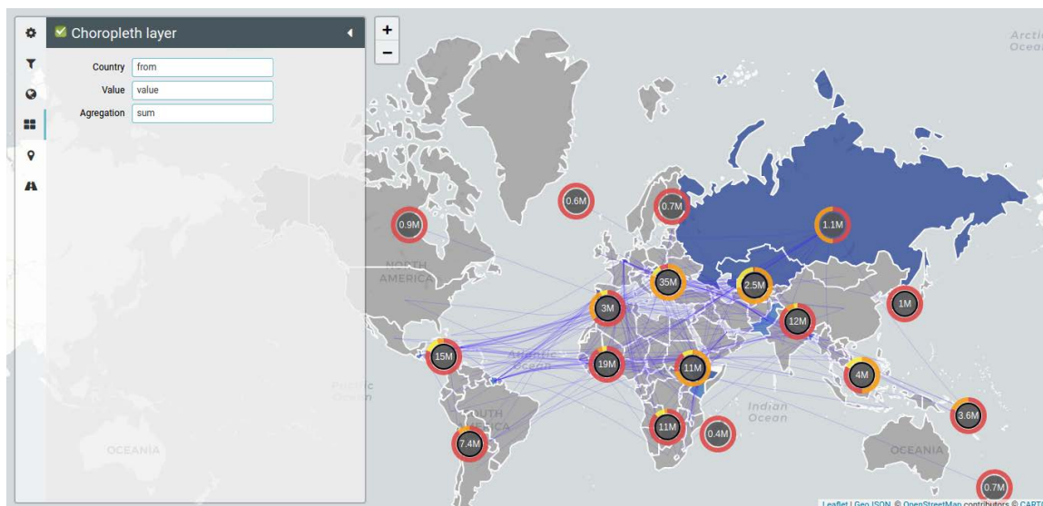
Obrázek 4.1: Ukázka rozhraní widgetu knihovny Geovisto zobrazující projekci více vrstev tematických map (zdroj: [17])
