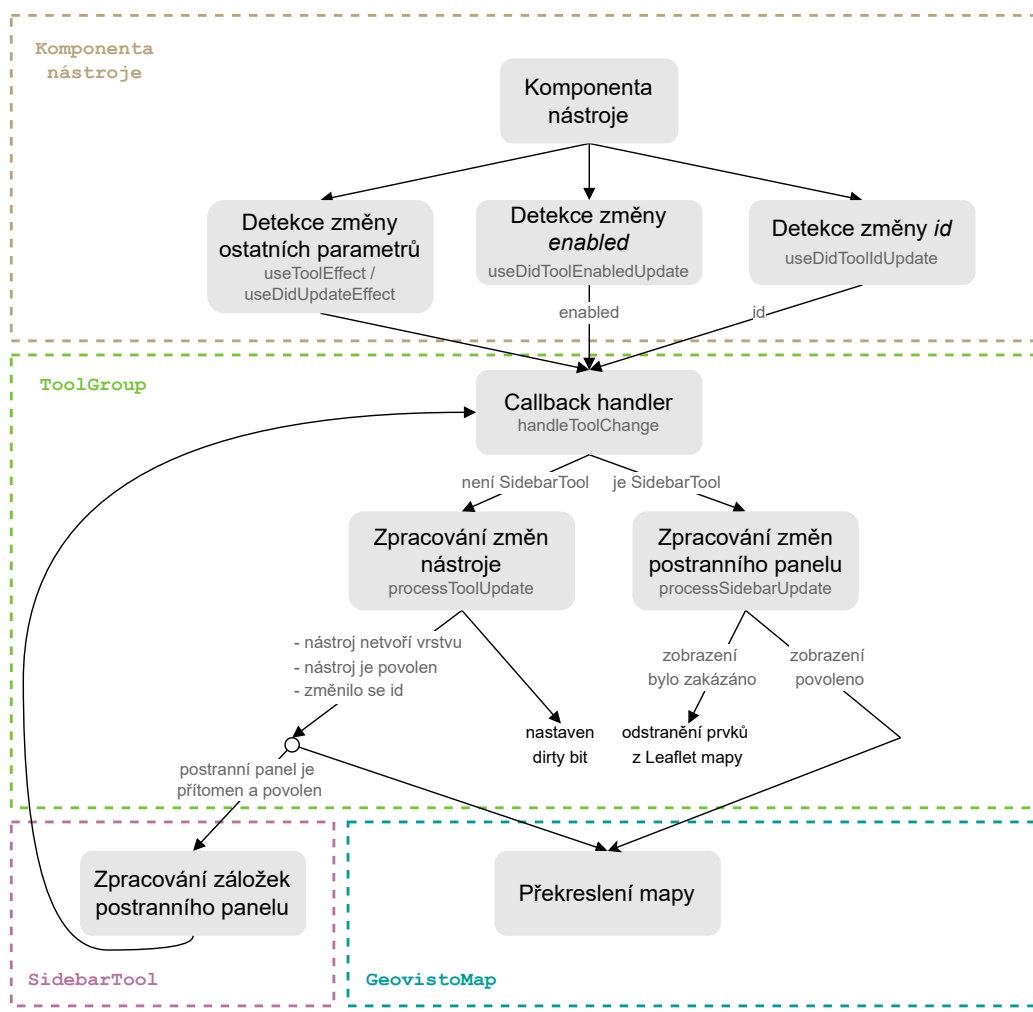
Obrázek 6.4: Předávání řízení při aktualizaci konfigurovatelných dat nástrojů 1
