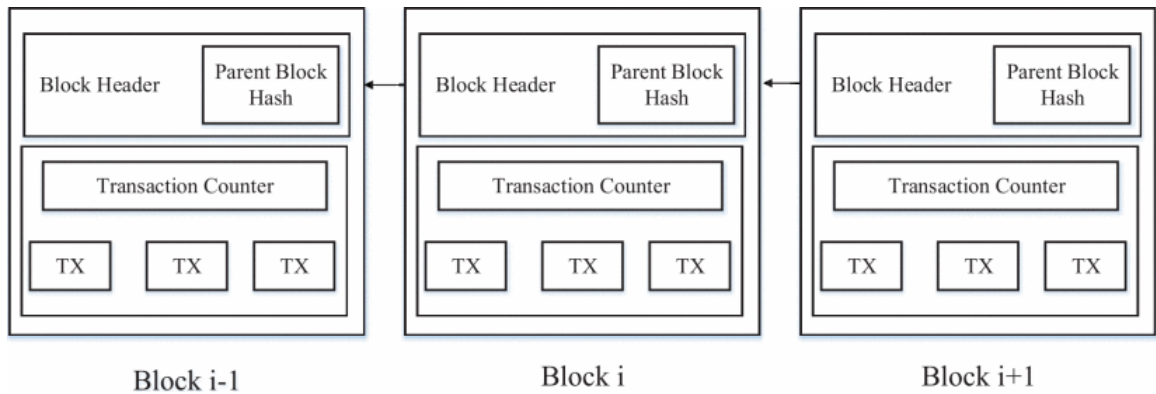
Obr. 3.2: Schéma blockchainu [23].
