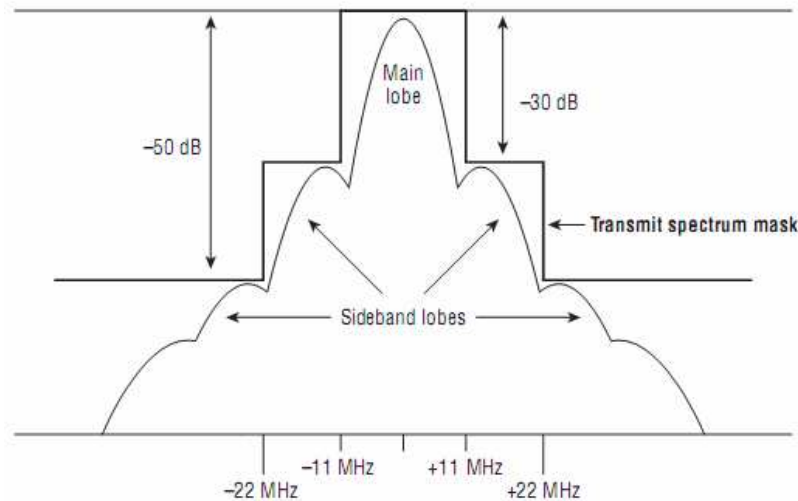
Obrázok 2.6.10: Vzhľad kanálového spektra na jednom kanále
