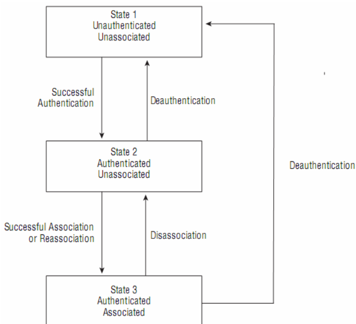
Obrázok 2.3.1: Postup asociácie a autentifikácie stanice s AP
