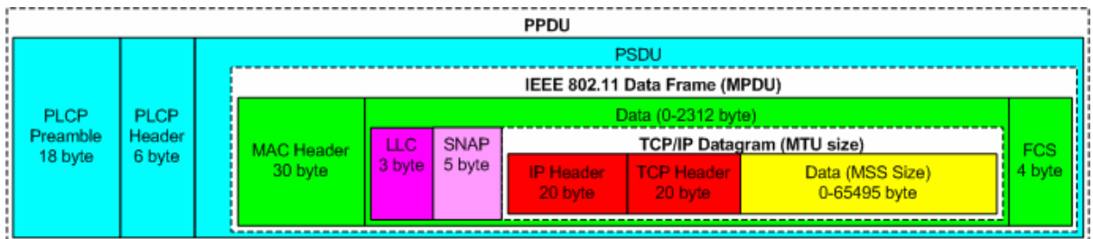
Obrázok 3.1.1: 802.11b/g paket
