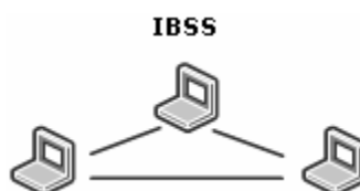
Obrázok 2.2.2: Ad-Hoc sieť
