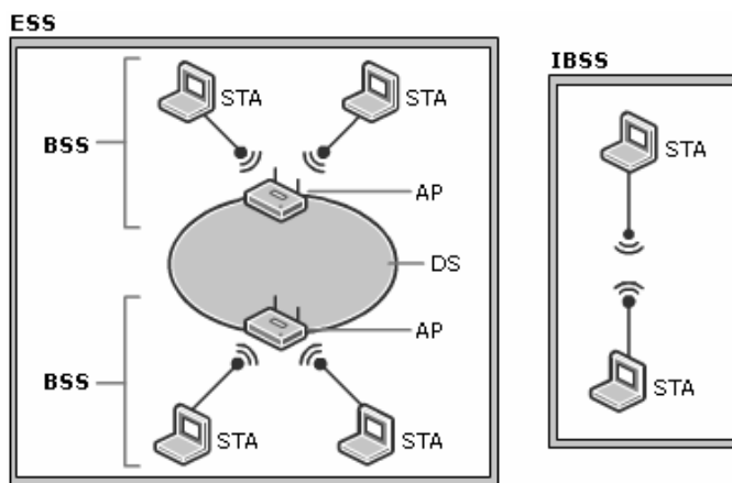
Obrázok 2.1: Architektúra sietí 802.11
