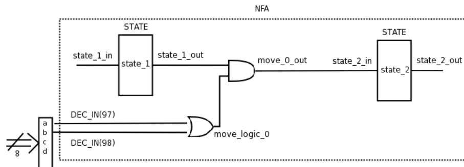
Obrázok 3.16: VHDL realizácia prechodu [ab]
