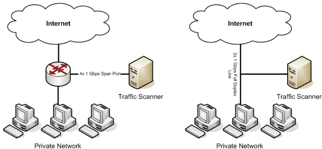
Obrázok 5.2: Sieťové zapojenie
