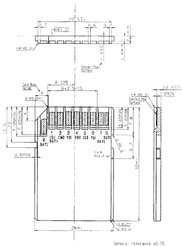
Obrázek 2.1: Rozměry SD karet
