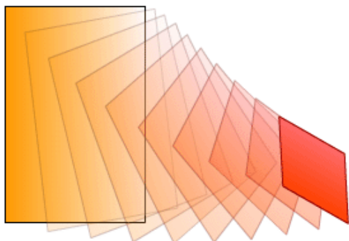
Obrázek 8a: MotionTween
