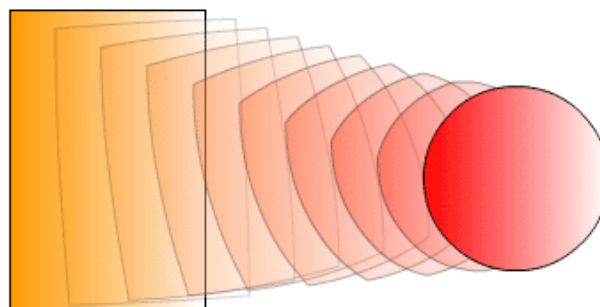
Obrázek 8b: ShapeTween
