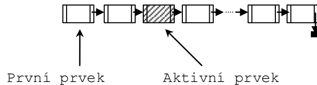
Obrázek 2: Jednosměrný seznam
