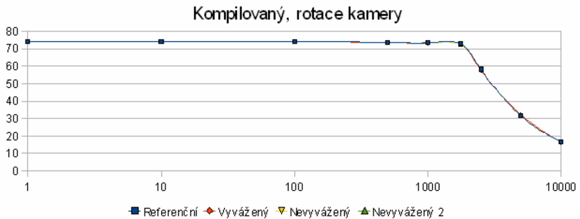
Graf 3.1: Ukázka výsledného grafu testování závislosti rozložení objektů v grafu scény při rotaci kamery a předkompilované větvi grafu na konfiguraci WinXP
