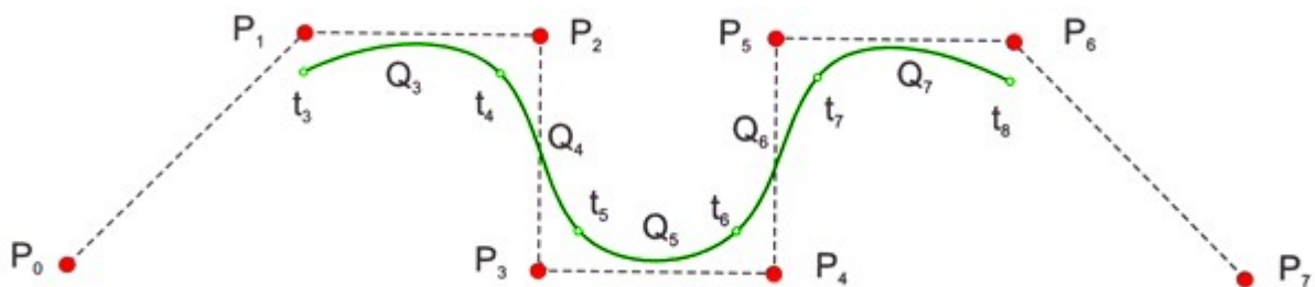
Obr. 4.5: Coonsův kubický B-spline
